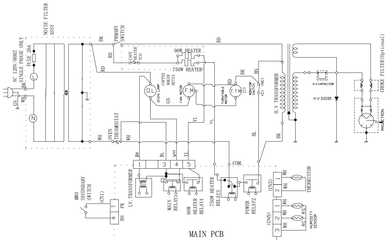
<Fig. 3. Schematic Diagram>
