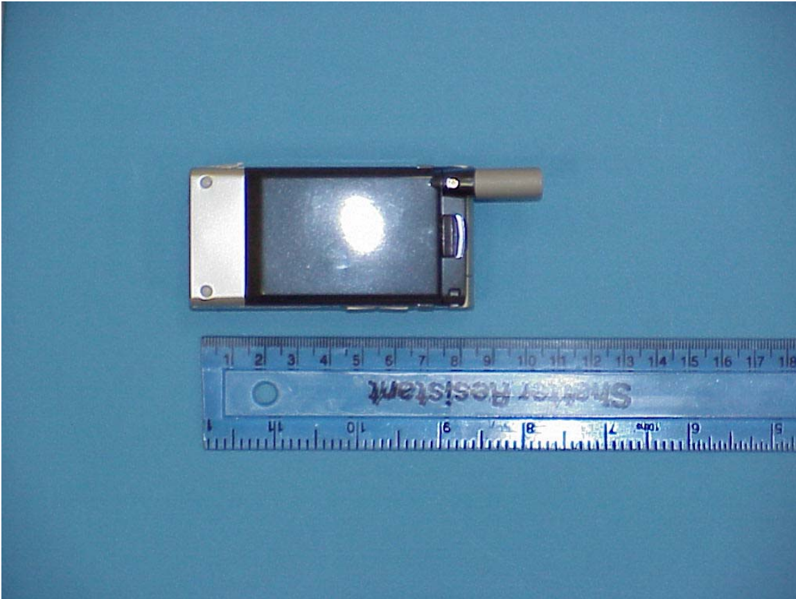
Photo 3 EUT back
