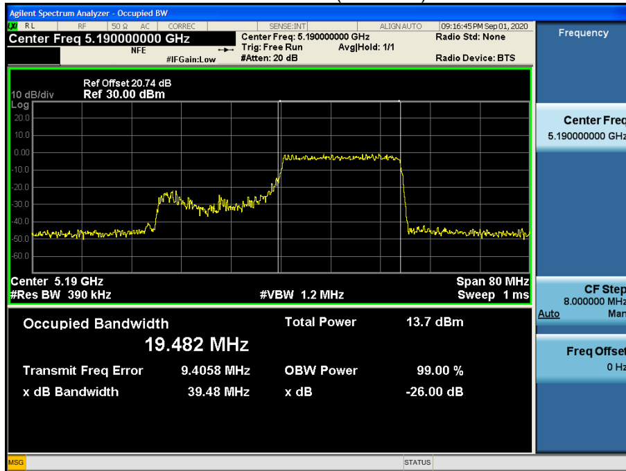
Bandwidth 40M Ch.38(5190MHz) RU 62
