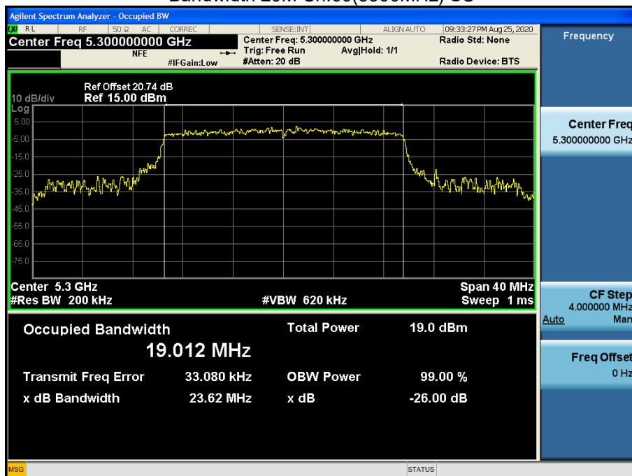
Bandwidth 20M Ch.60(5300MHz) SU
