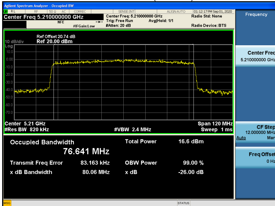
Bandwidth 80M Ch.42(5210MHz) SU
