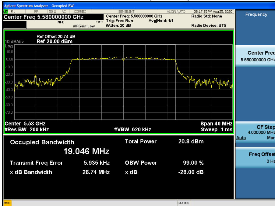
Bandwidth 20M Ch.116(5580MHz) RU 61
