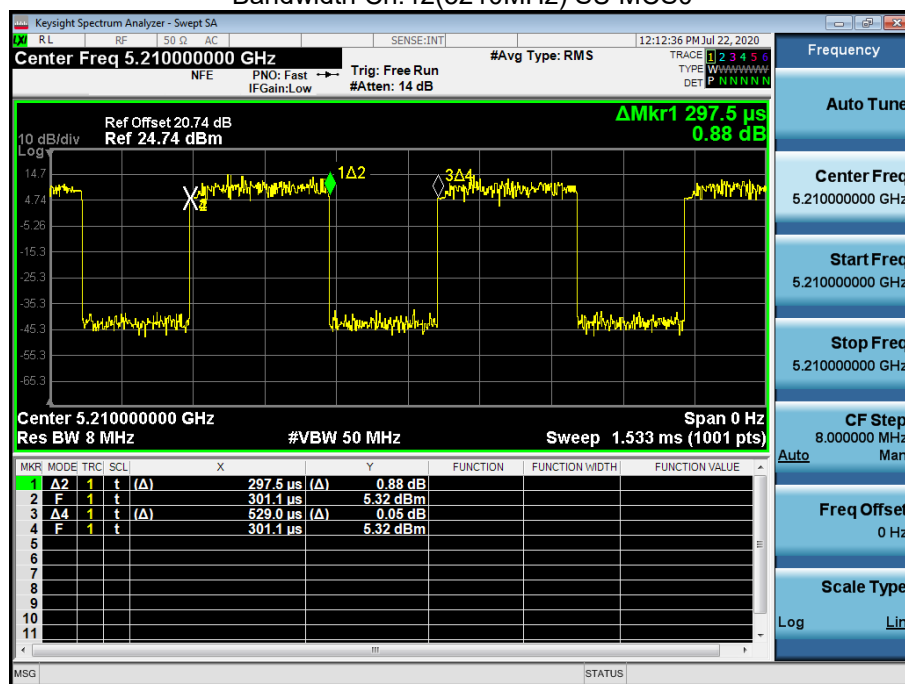
Bandwidth Ch.42(5210MHz) SU MCS0
