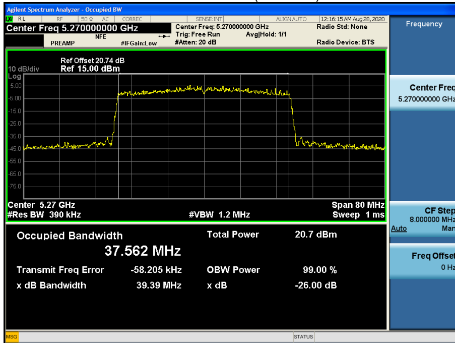
Bandwidth 40M Ch.54(5270MHz) SU
