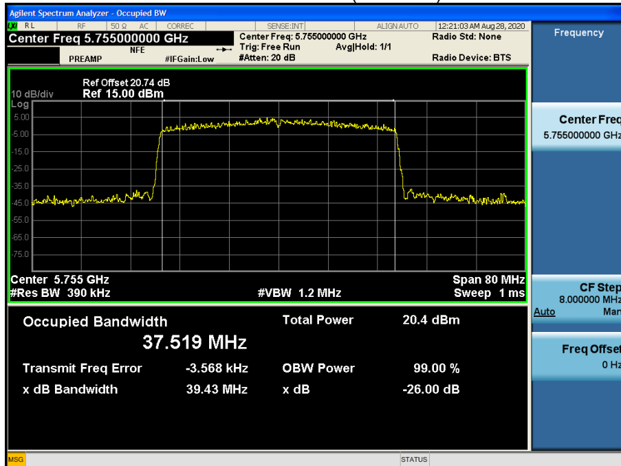
Bandwidth 40M Ch.151(5755MHz) SU
