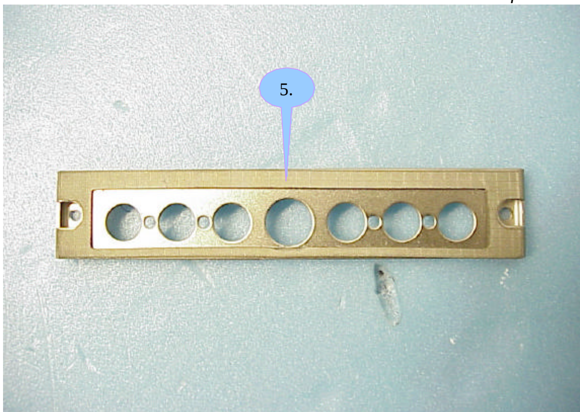
Figure 30 Bracket of AV and Component Jacks
