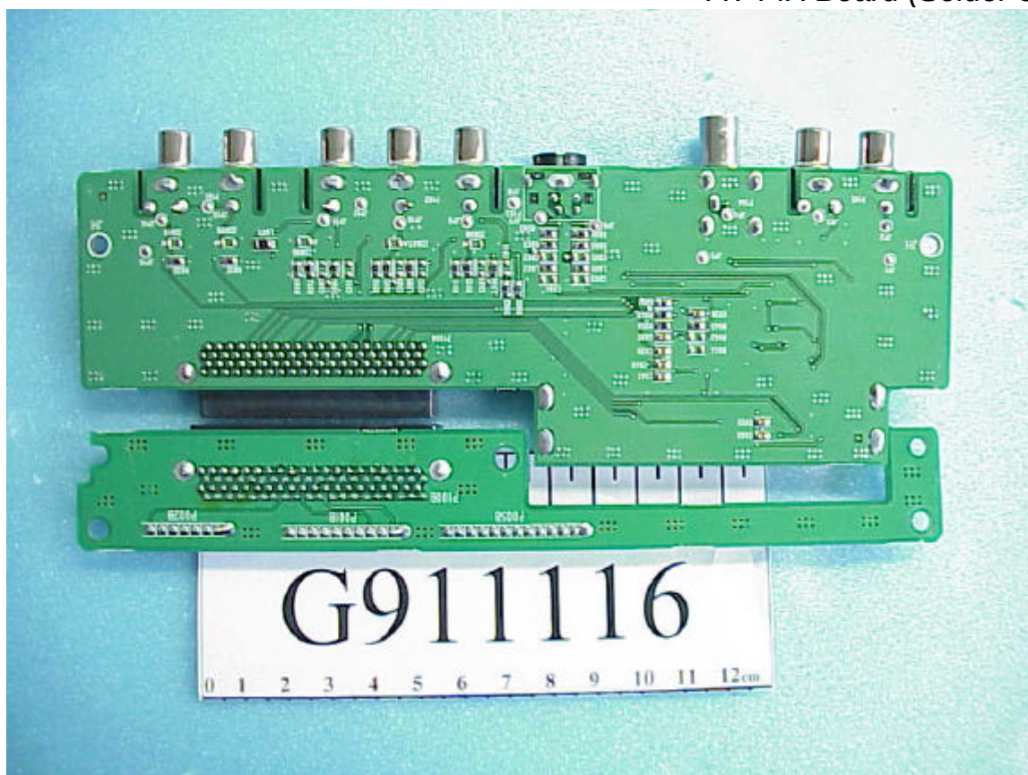
Figure 14 AV FIX Board (Solder Side)
