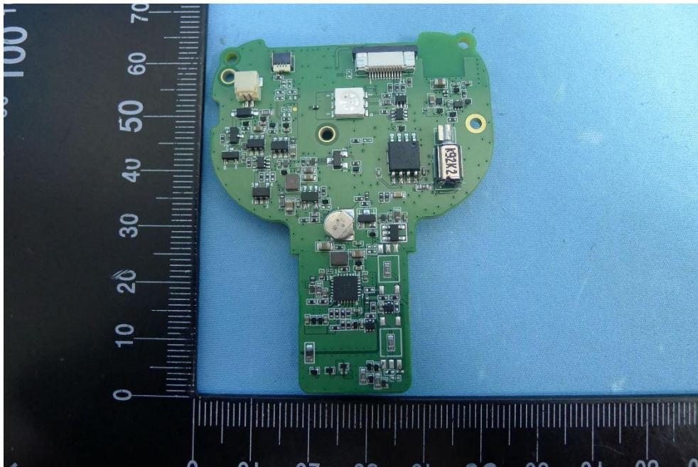
(8) EUT Photo (MS852B)
