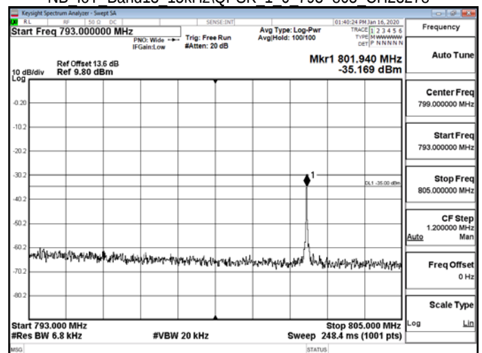
NB IoT Band13 15kHz/QPSK 1 0 793-805 CH23278
