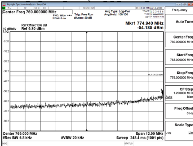
NB IoT Band13 15kHz/QPSK 1 0 793-805 CH23182
