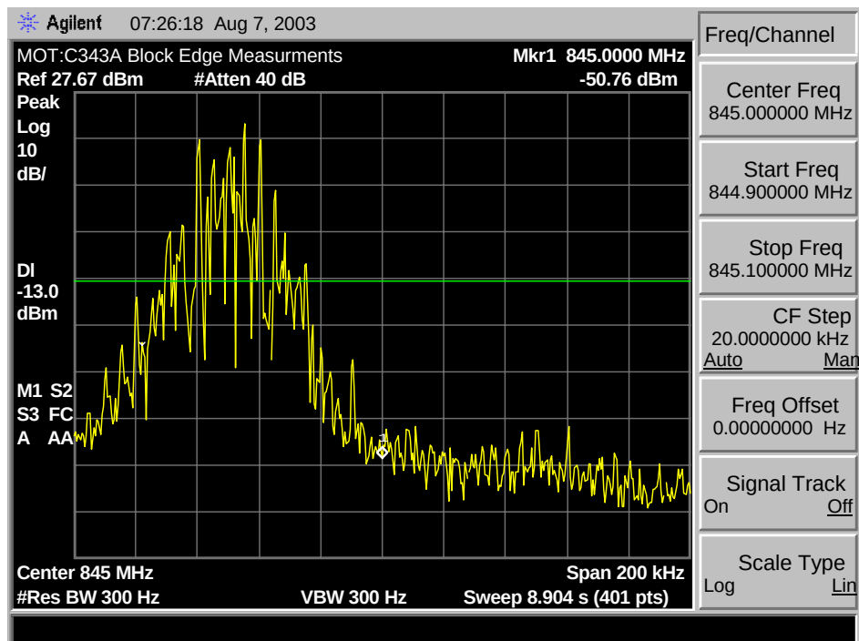
800 AMPS B Max/A* (Upper) Min. Block Edge
