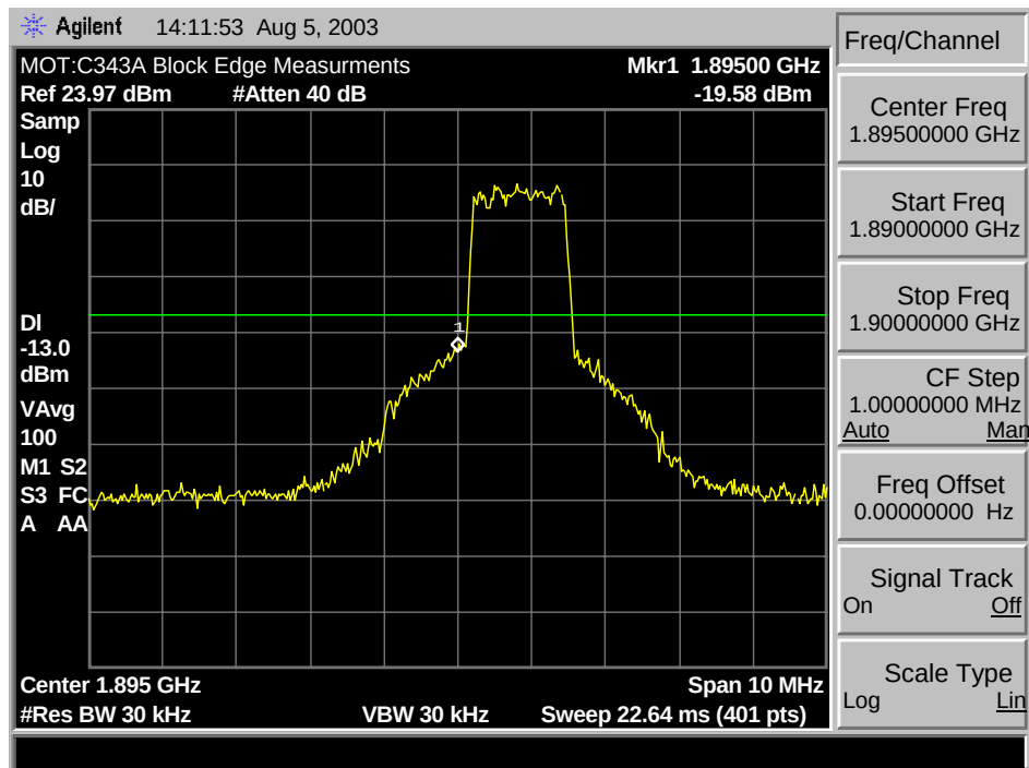
1900 CDMA C, C2, C3 Min. Block Edge
