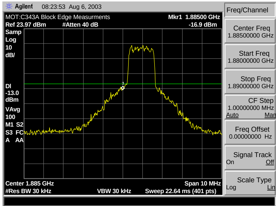
1900 CDMA E Min. Block Edge
