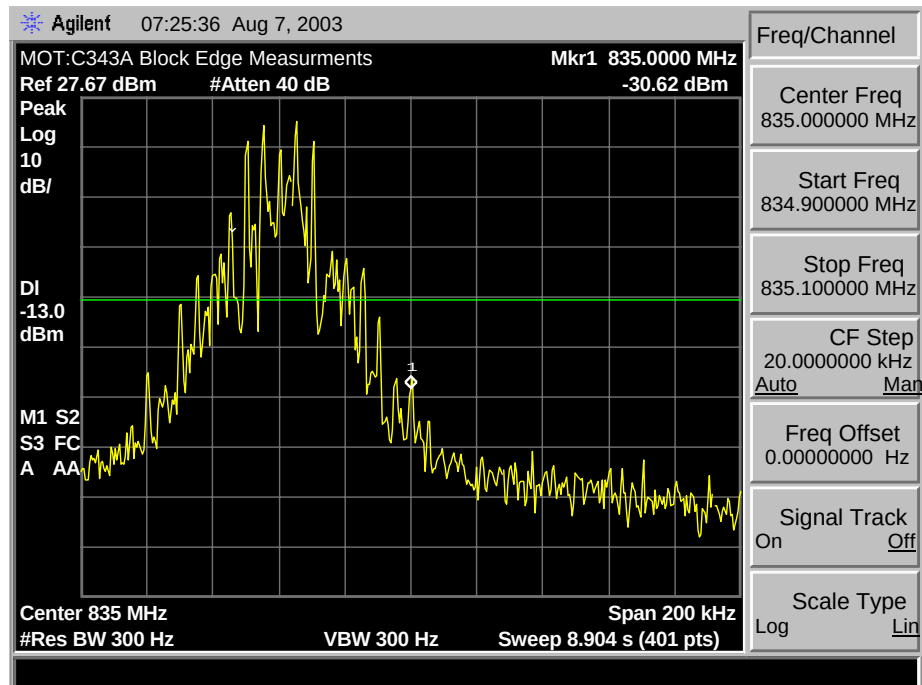
800 AMPS A Max/B Min. Block Edge
