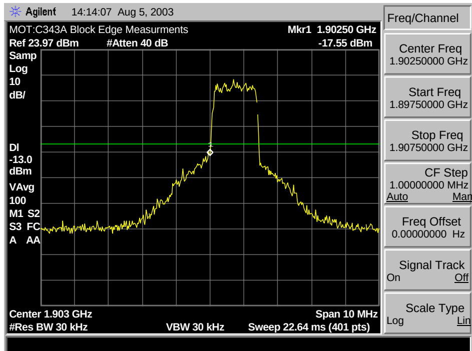
1900 CDMA C1 Min. Block Edge
