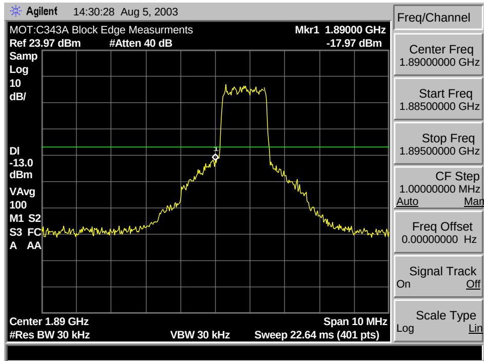
1900 CDMA F Min. Block Edge
