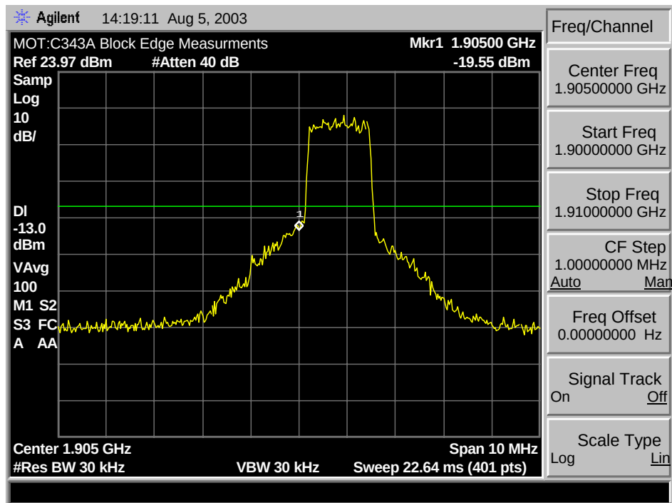
1900 CDMA C5 Min. Block Edge
