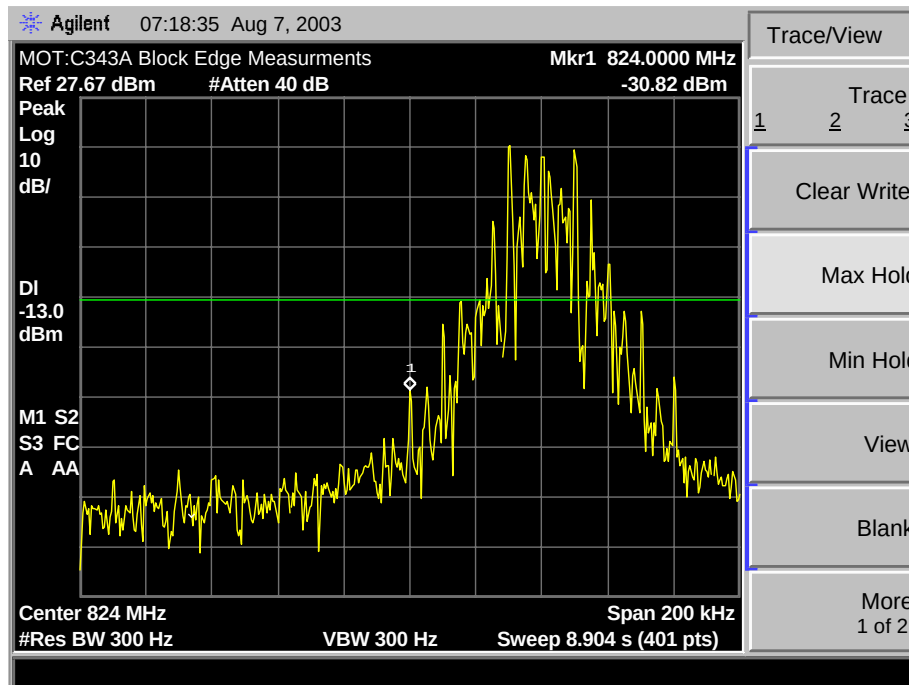
800 AMPS A*(Lower) Min. Block Edge
