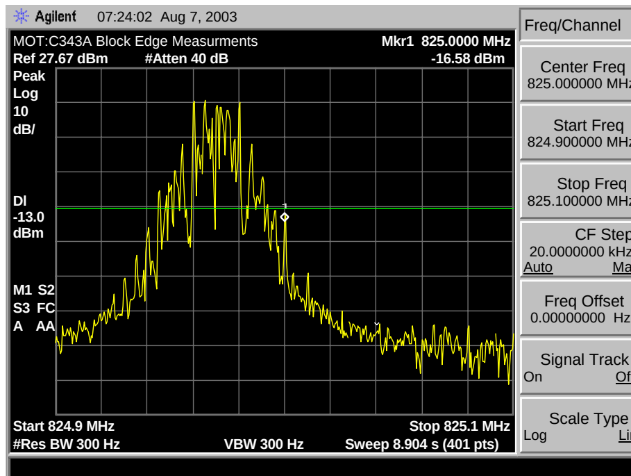
800 AMPS A*(Lower) Max/A Min. Block Edge
