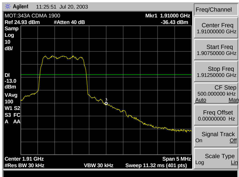
1900 CDMA Upper Band Edge
