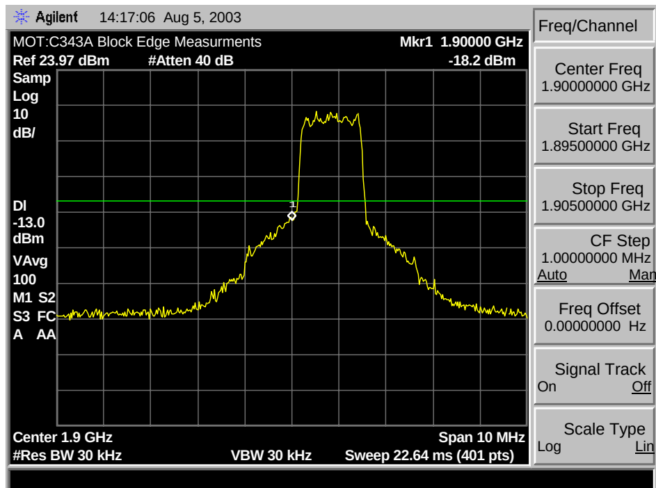
1900 CDMA C4 Min. Block Edge
