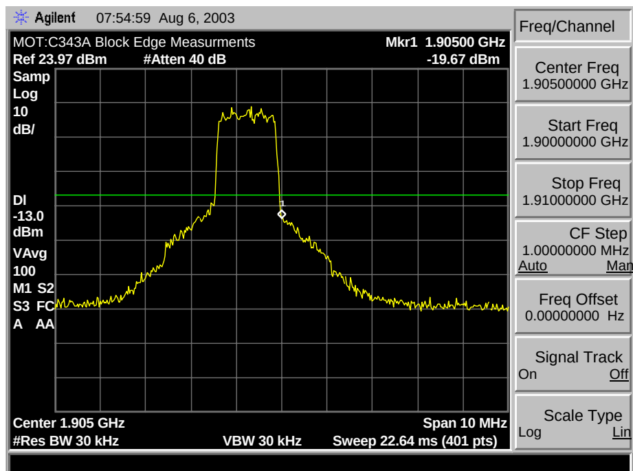
1900 CDMA C4 Max. Block Edge
