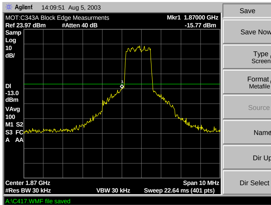
1900 CDMA B Min. Block Edge
