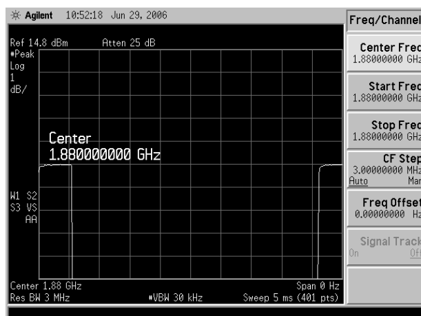
GSM 1880 MHz
