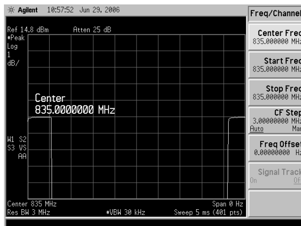
GSM 835 MHz
