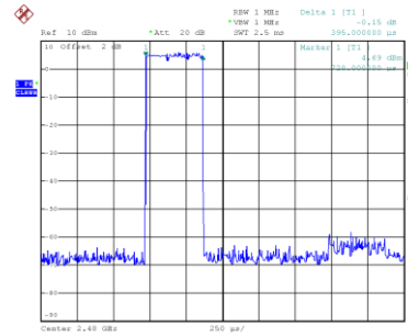
CH78-3DH1
