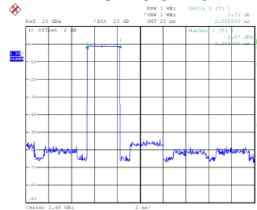
CH78-3DH5
