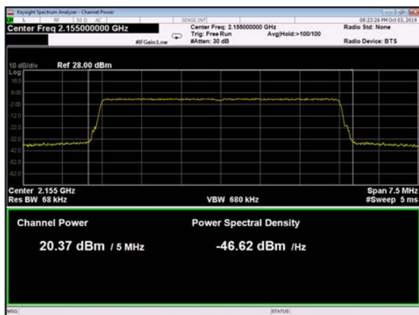
Figure 50 5MHz BW, 2155MHz
