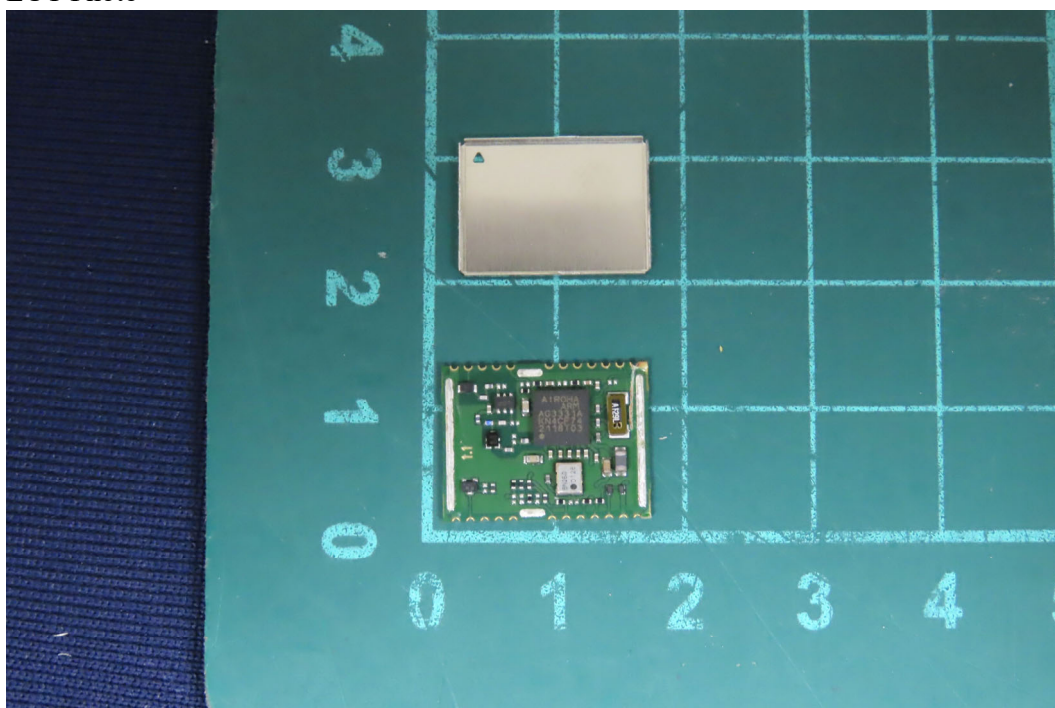
(15) EUT Photo
