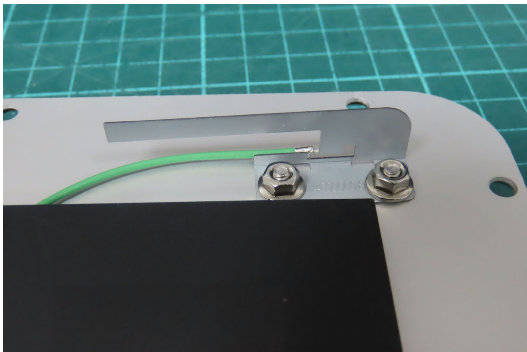
(24) EUT Photo
