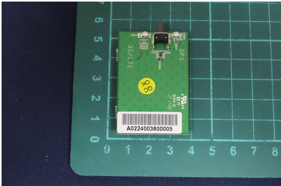
(6) EUT Photo
