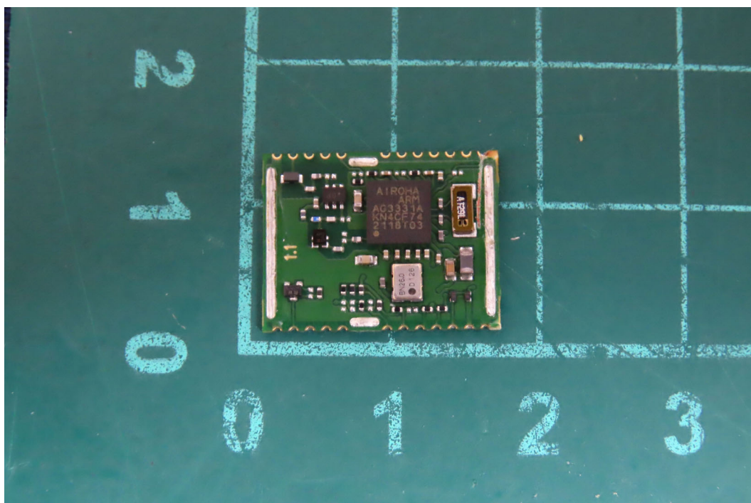
(16) EUT Photo
