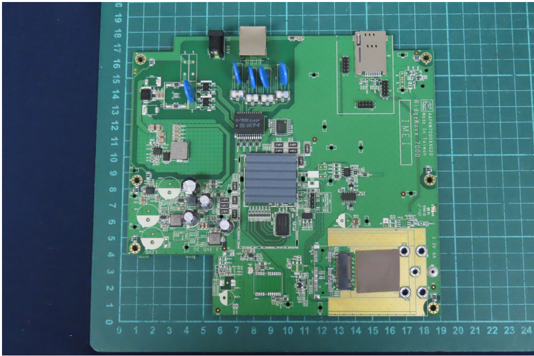
(18) EUT Photo
