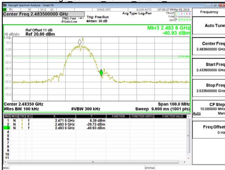
Band Edge 802.11b 20MHz Chain0 2472MHz
