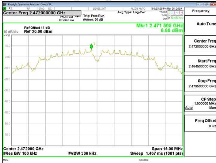
Reference Level 802.11b 20MHz Chain0 2472MHz
