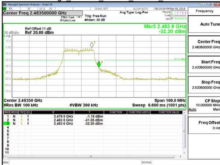
Band Edge 802.11n 20MHz Chain0 2472MHz
