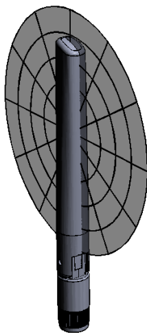
YZ-Plane Gain
