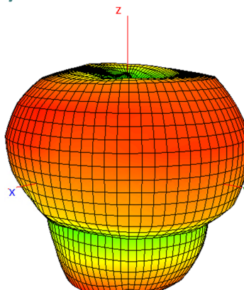
2450 MHz
