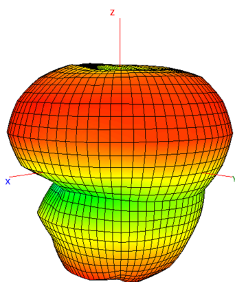
2400 MHz
