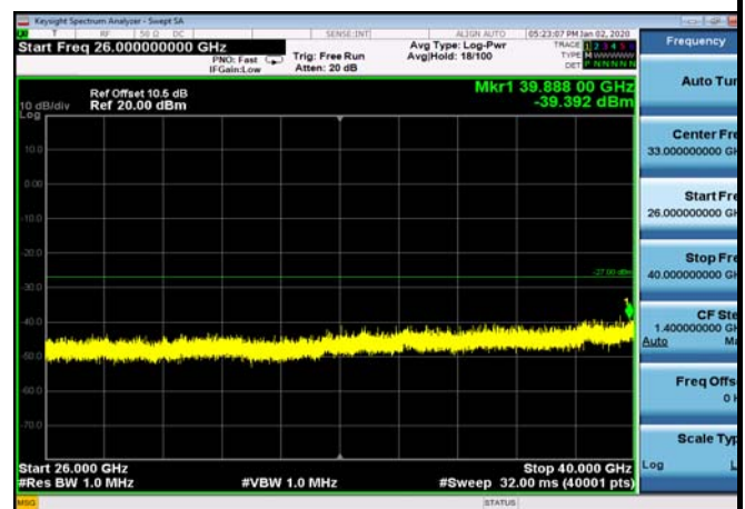
U-NII-1 ,Plot 4,26000MHz~40000MHz-802. 11ac(40MHz),5230MHz,Ant1
