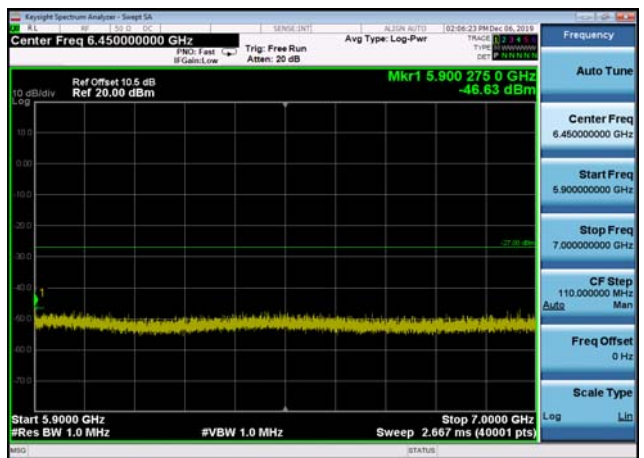
U-NII-3 ,Plot 3,5900MHz~7000MHz-802.1 1n(40MHz),5795MHz,Ant1
