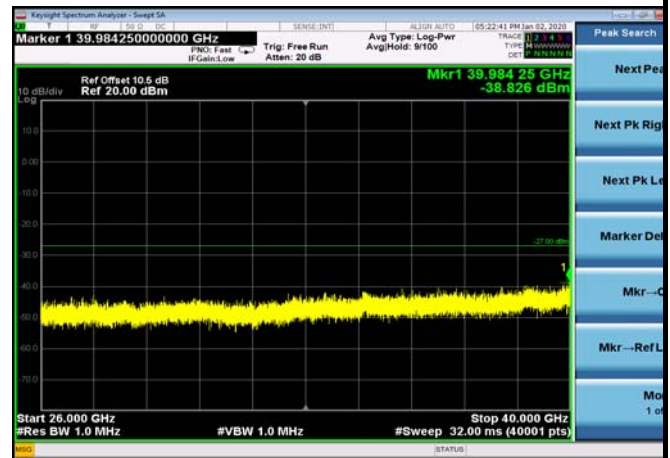
U-NII-1 ,Plot 4,26000MHz~40000MHz-802. 11ac(20MHz),5220MHz,Ant1
