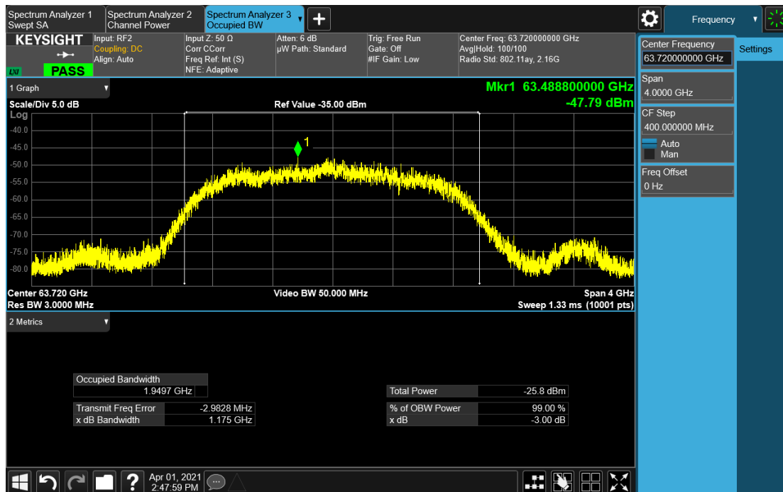
Wave-AP_2GHz_63.72GHz_Peak
