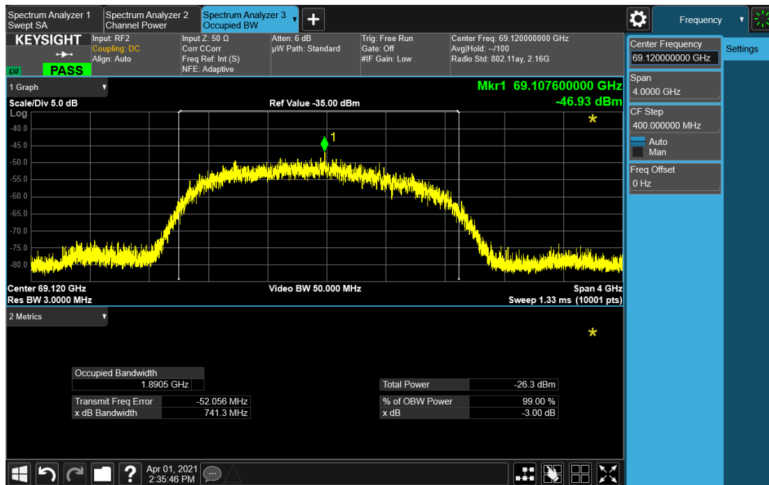
Wave-AP_2GHz_69.12GHz_Peak
