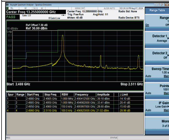
Band41_15MHz_QPSK_39725_1RB#0
