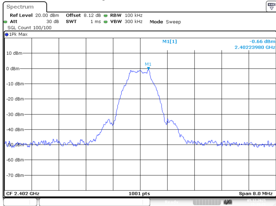
Band Edge NVNT GFSK 2402MHz Ant1 Ref
