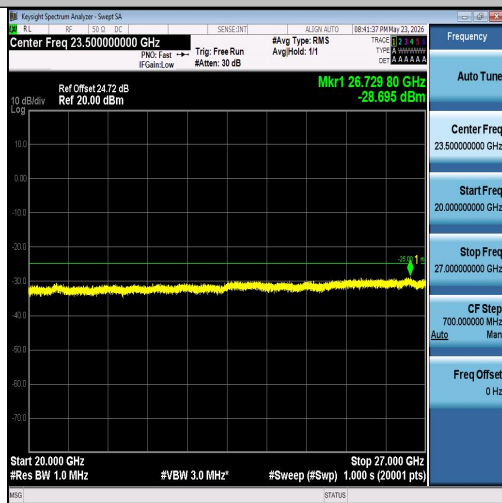
Band7-10MHz-QPSK-21400-50RB#0-20000~27
