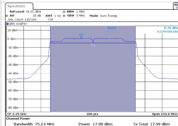
MIMO A-802.11ac80-80MHz-Ch58-5290MHz-VHT0
