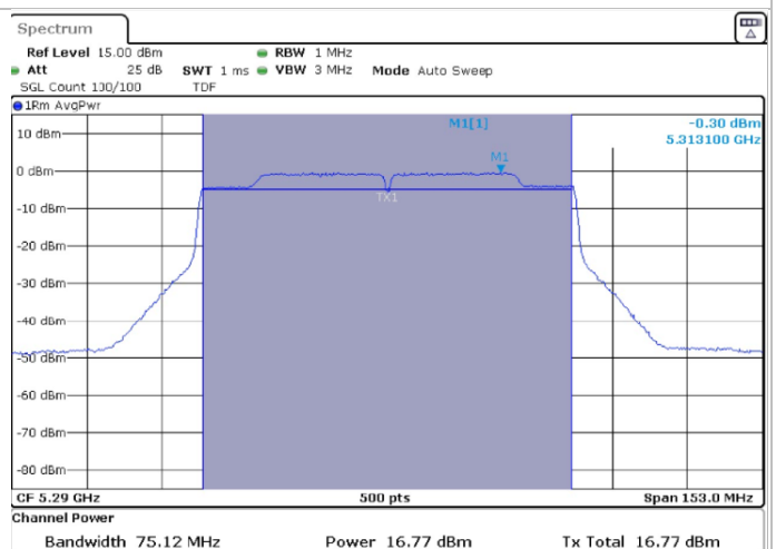
MIMO B-802.11ac-80MHz-Ch58-5290MHz-VHT0
