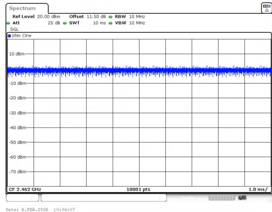
IEEE 802.11g_20MHz_Channel 11
