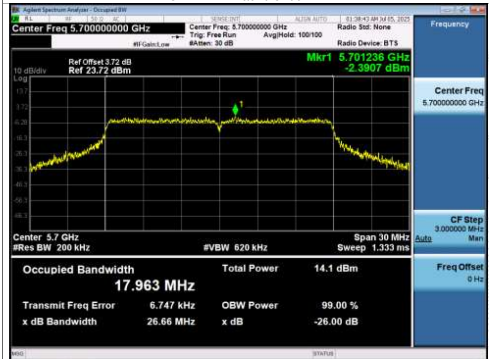
OBW NVNT ac20 5700MHz
