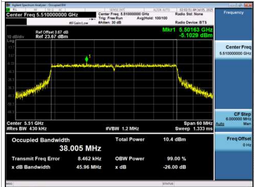
OBW NVNT ax40 5510MHz
