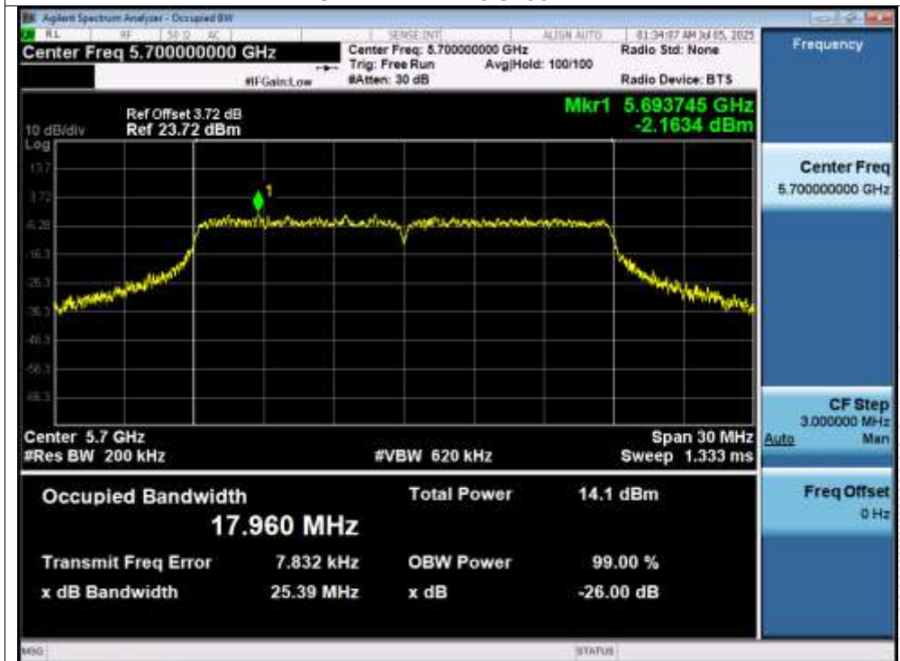
OBW NVNT n20 5700MHz
