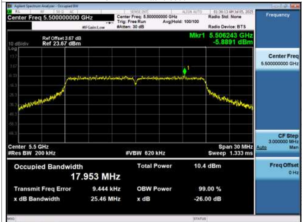
OBW NVNT ac20 5500MHz
