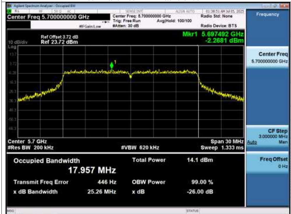
-26dB Bandwidth NVNT ac20 5700MHz
