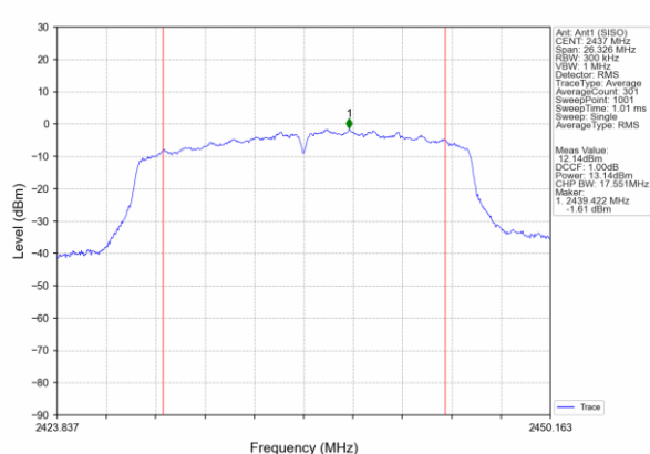
2437MHz
