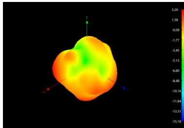
2500MHz
