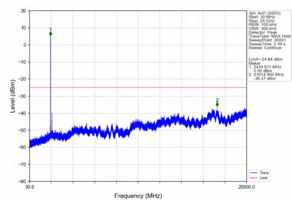
802.11b_MCH_2437MHz_Ant1 (SISO)_NTNV
