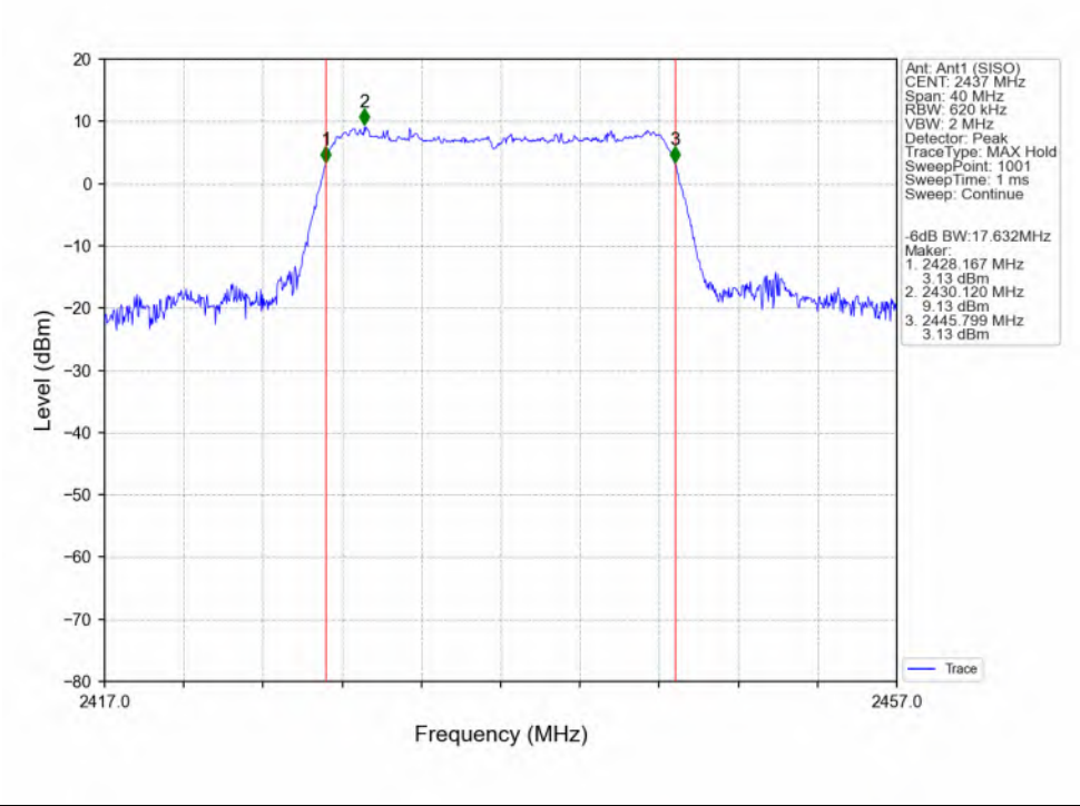
802.11n(HT20)_MCH_2437MHz_Ant1 (SISO)_NTNV
