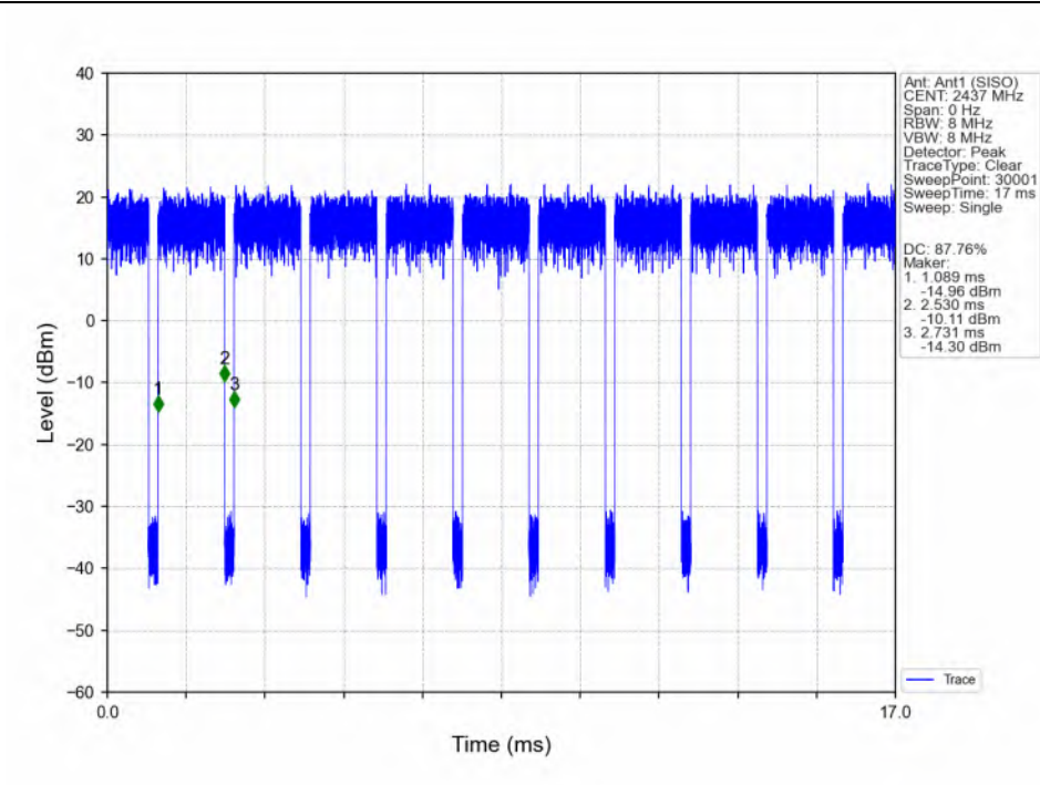
802.11g_MCH_2437MHz_Ant1 (SISO)_NTNV
