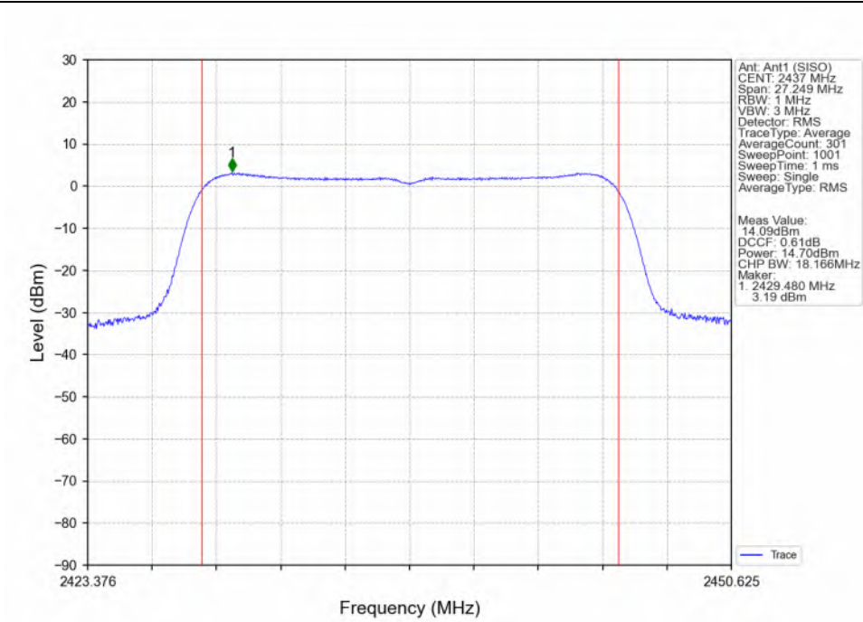
802.11n(HT20)_MCH_2437MHz_Ant1 (SISO)_NTNV
