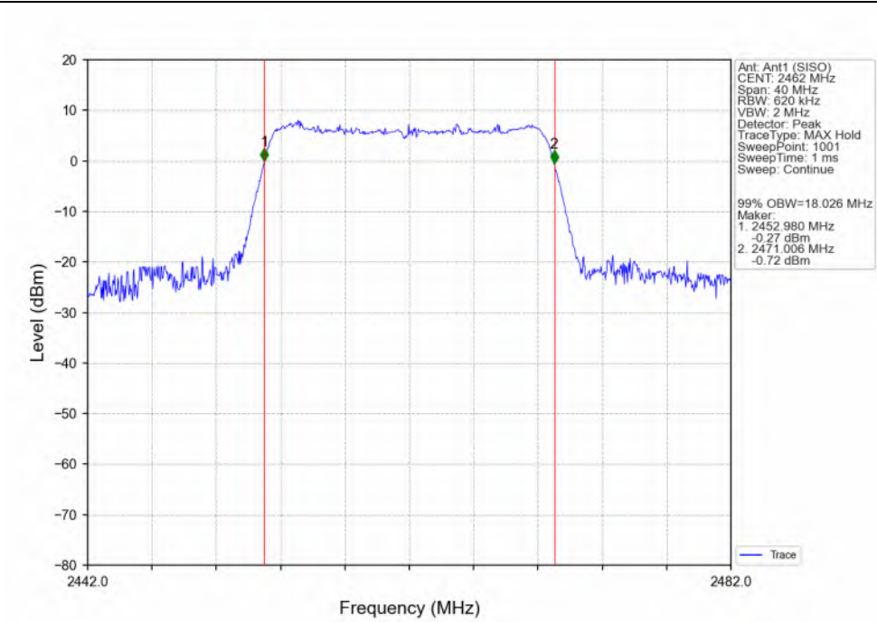
802.11n(HT20)_HCH_2462MHz_Ant1 (SISO)_NTNV
