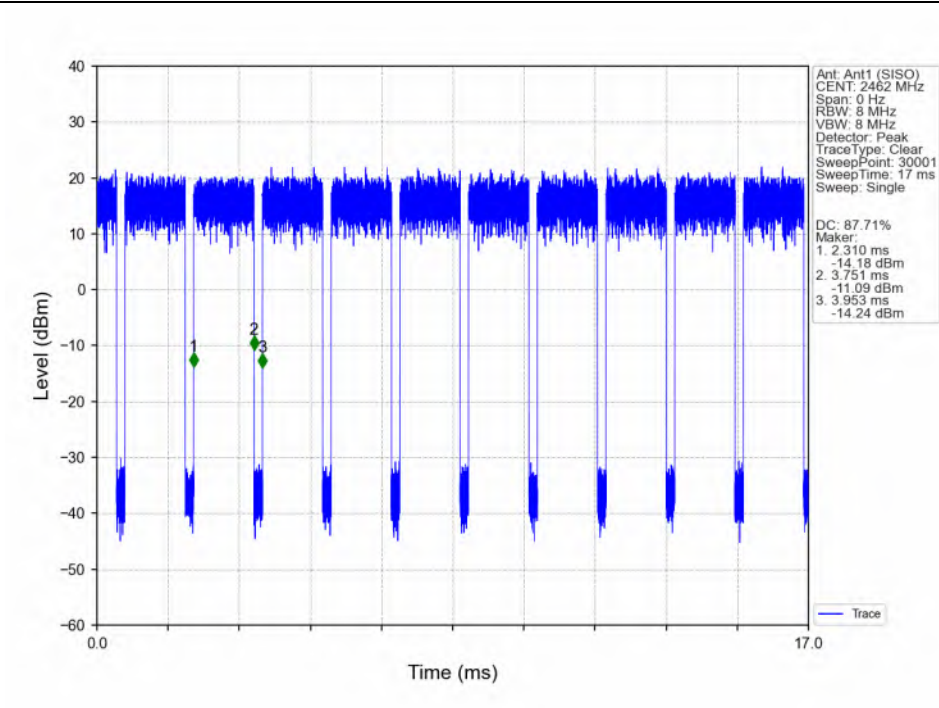
802.11g_HCH_2462MHz_Ant1 (SISO)_NTNV
