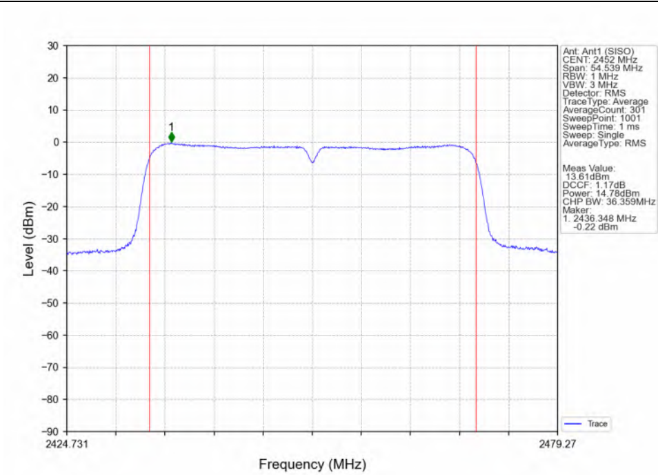
802.11n(HT40)_HCH_2452MHz_Ant1 (SISO)_NTNV
