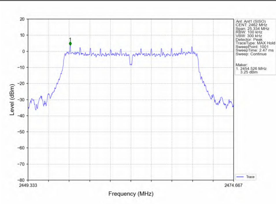
802.11g_HCH_2462MHz_Ant1 (SISO)_NTNV
