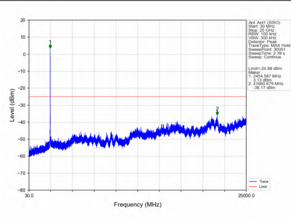
802.11g_HCH_2462MHz_Ant1 (SISO)_NTNV
