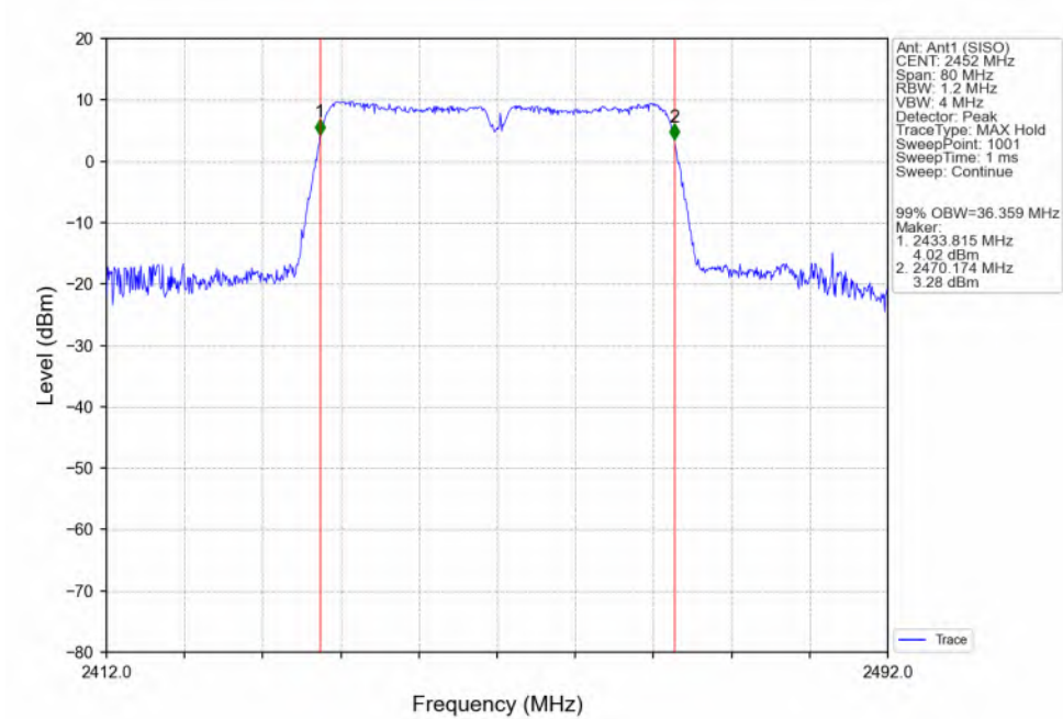
802.11n(HT40)_HCH_2452MHz_Ant1 (SISO)_NTNV
