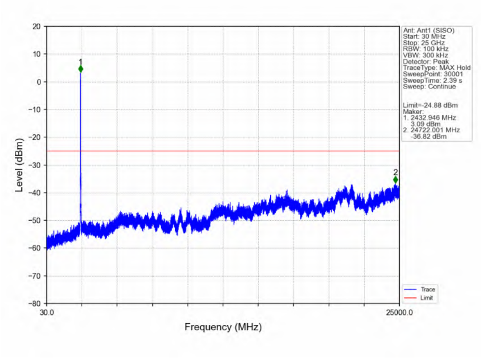
802.11g_MCH_2437MHz_Ant1 (SISO)_NTNV
