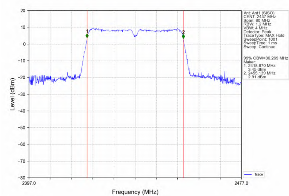
802.11n(HT40)_MCH_2437MHz_Ant1 (SISO)_NTNV
