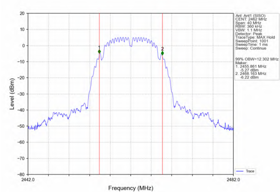
802.11b_HCH_2462MHz_Ant1 (SISO)_NTNV
