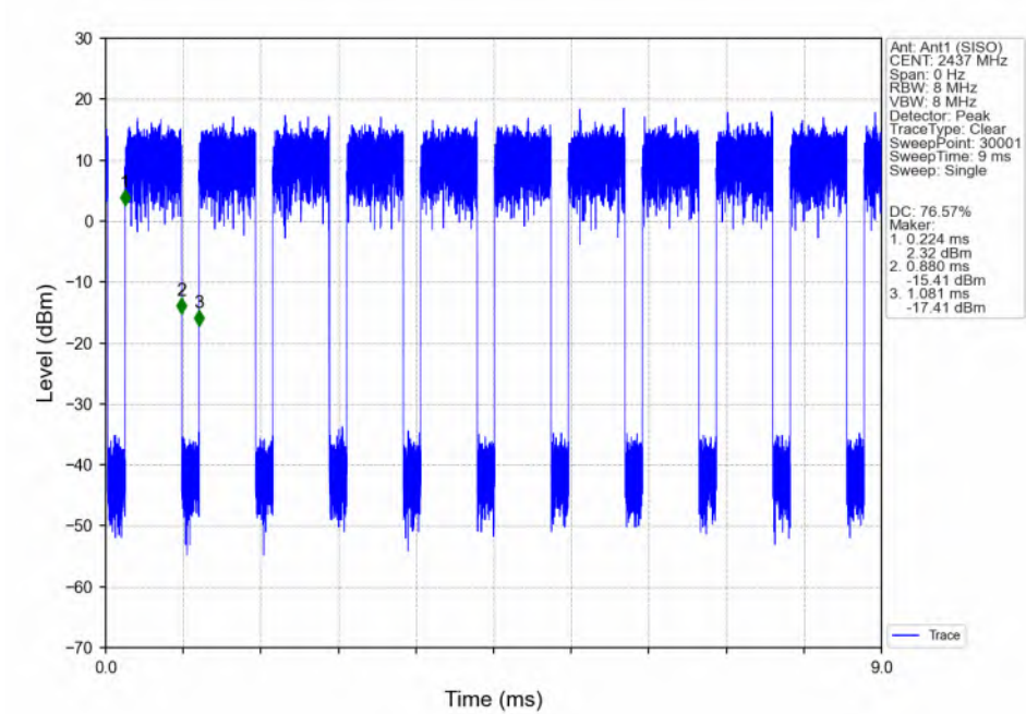
802.11n(HT40)_MCH_2437MHz_Ant1 (SISO)_NTNV
