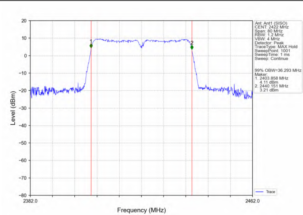
802.11n(HT40)_LCH_2422MHz_Ant1 (SISO)_NTNV
