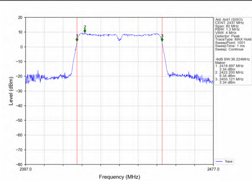
802.11n(HT40)_MCH_2437MHz_Ant1 (SISO)_NTNV
