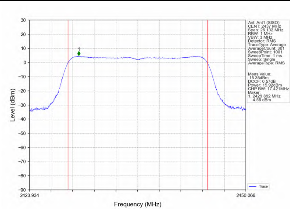
802.11g_MCH_2437MHz_Ant1 (SISO)_NTNV
