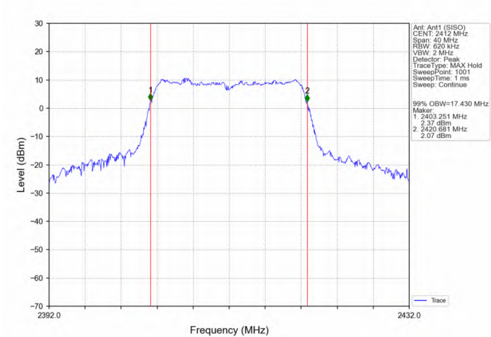
802.11g_LCH_2412MHz_Ant1 (SISO)_NTNV
