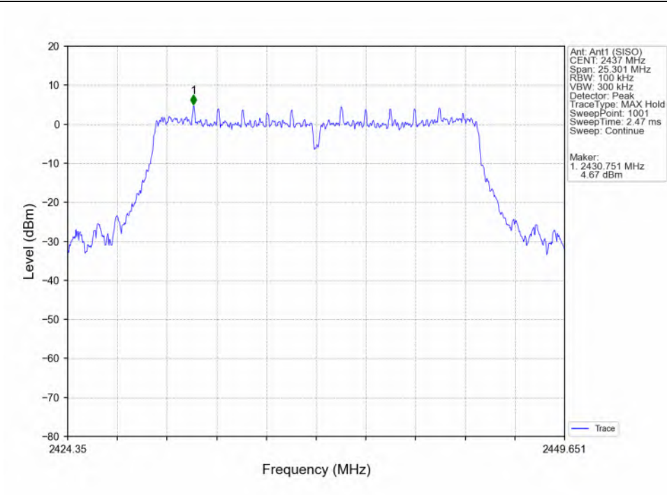
802.11g_MCH_2437MHz_Ant1 (SISO)_NTNV
