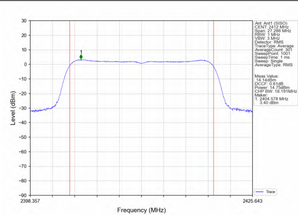
802.11n(HT20)_LCH_2412MHz_Ant1 (SISO)_NTNV
