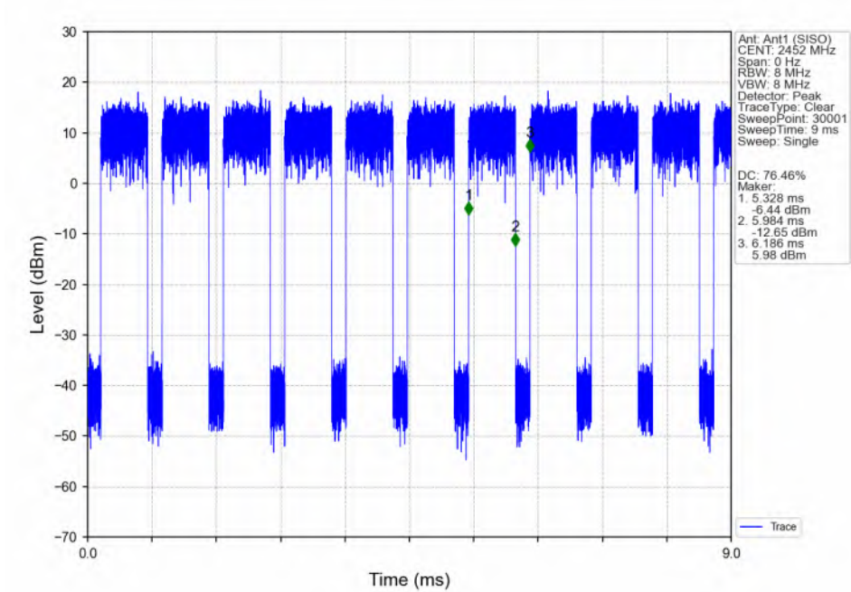
802.11n(HT40)_HCH_2452MHz_Ant1 (SISO)_NTNV
