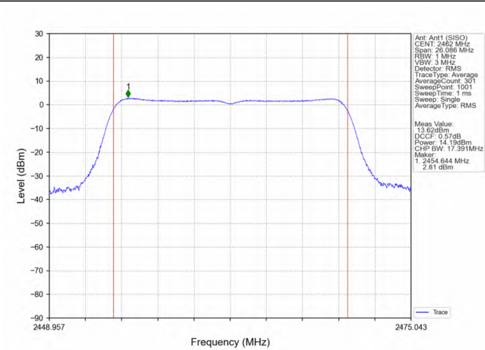
802.11g_HCH_2462MHz_Ant1 (SISO)_NTNV
