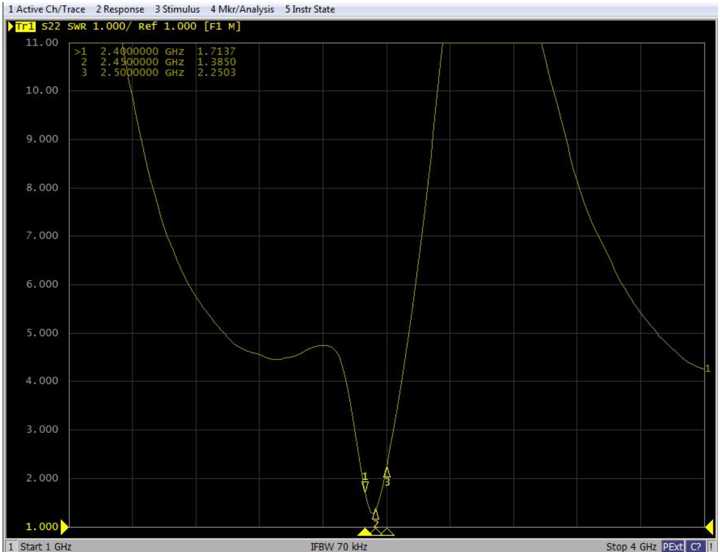
F600 antenna VSWR
