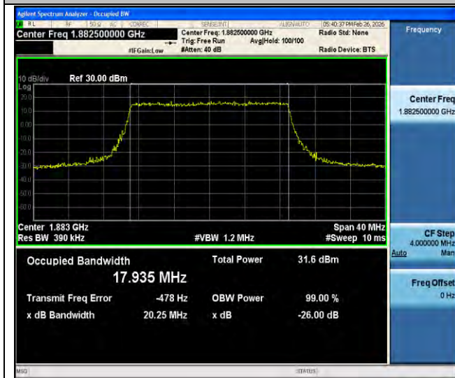
Band25-20MHz-QPSK-26365-100RB#0-PASS
