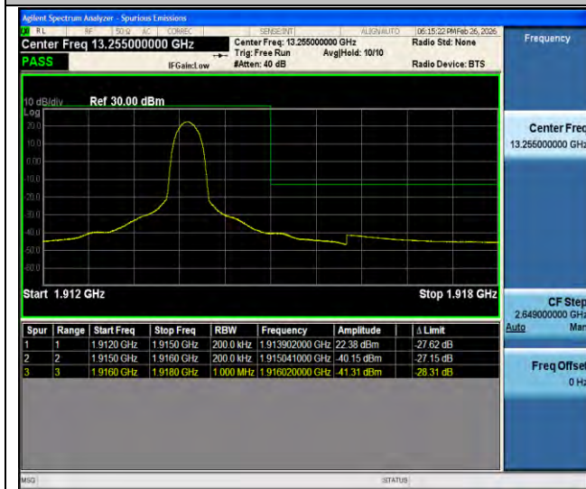
Band25-20MHz-QPSK-26590-1RB#99-PASS
