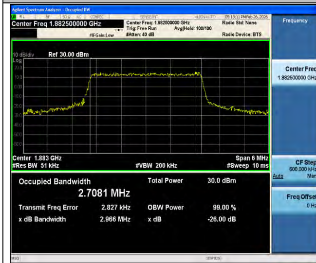
Band25-3MHz-QPSK-26365-15RB#0-PASS
