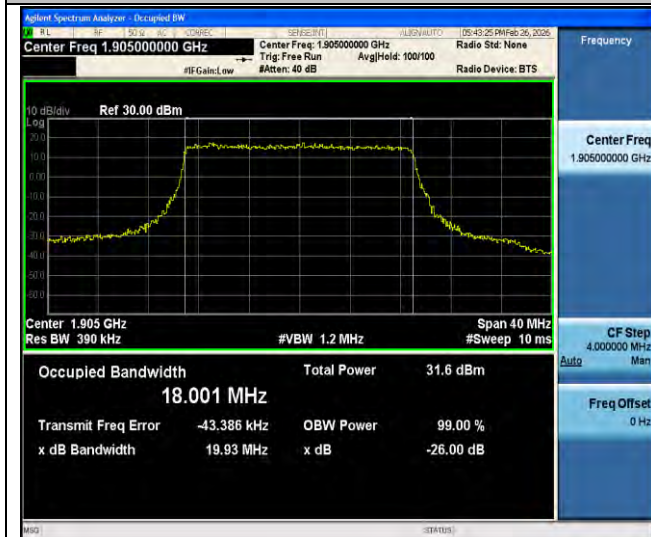
Band25-20MHz-QPSK-26590-100RB#0-PASS
