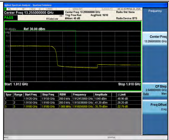
Band25-20MHz-QPSK-26590-100RB#0-PASS
