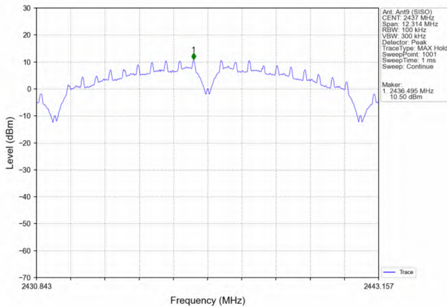
802.11b_MCH_2437MHz_Ant9 (SISO)_NTNV
