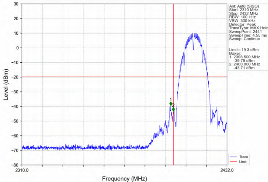
802.11b_LCH_2412MHz_Ant8 (SISO)_NTNV
