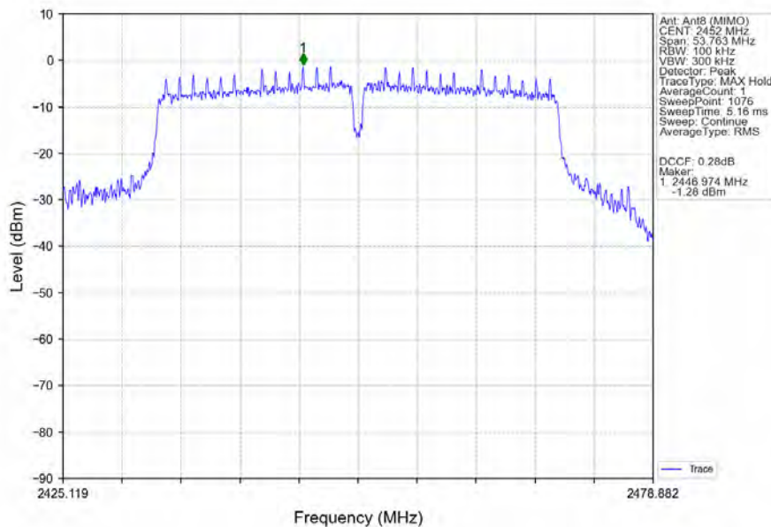
802.11n(HT40)_HCH_2452MHz_Ant8 (MIMO)_NTNV
