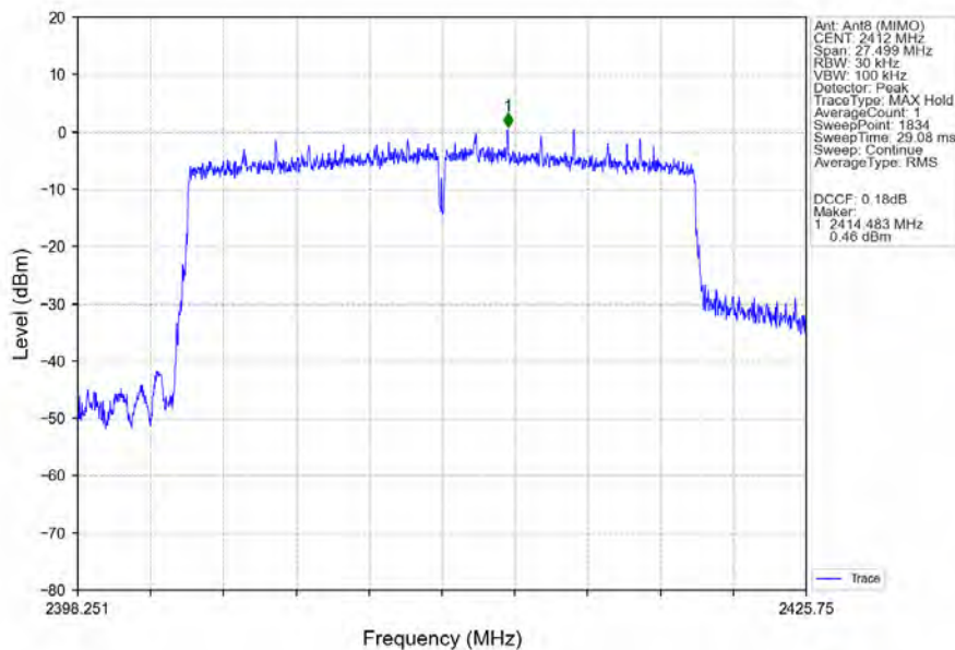
802.11ax(HEW20)_LCH_2412MHz_RU242_Left_Ant8 (MIMO)_NTNV
