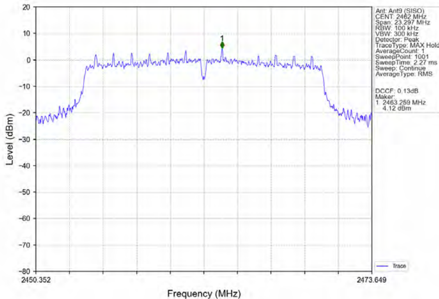
802.11g_HCH_2462MHz_Ant9 (SISO)_NTNV
