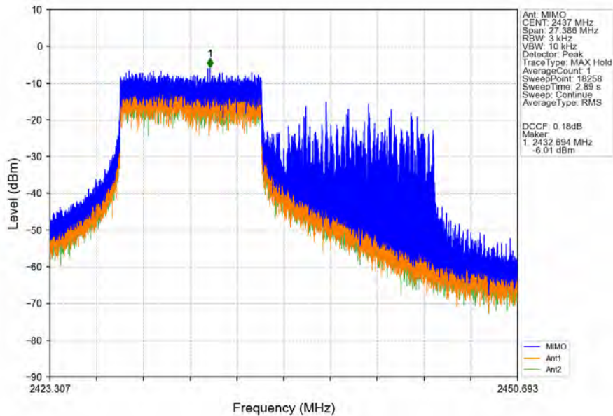
802.11ax(HEW20)_MCH_2437MHz_RU242_Left_Ant8 (MIMO)_NTNV
