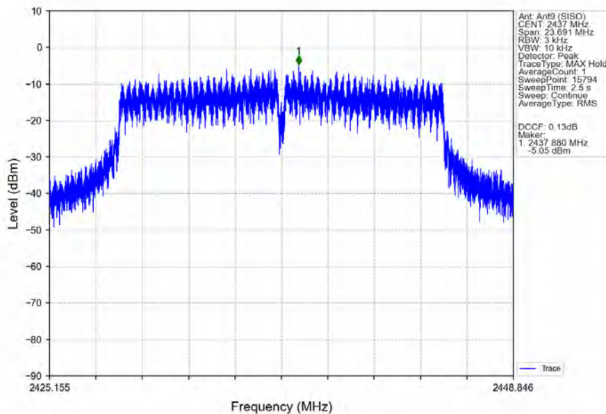
802.11g_MCH_2437MHz_Ant9 (SISO)_NTNV
