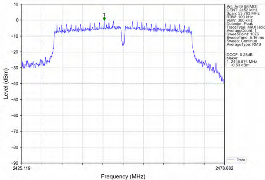
802.11n(HT40)_HCH_2452MHz_MIMO_NTNV
