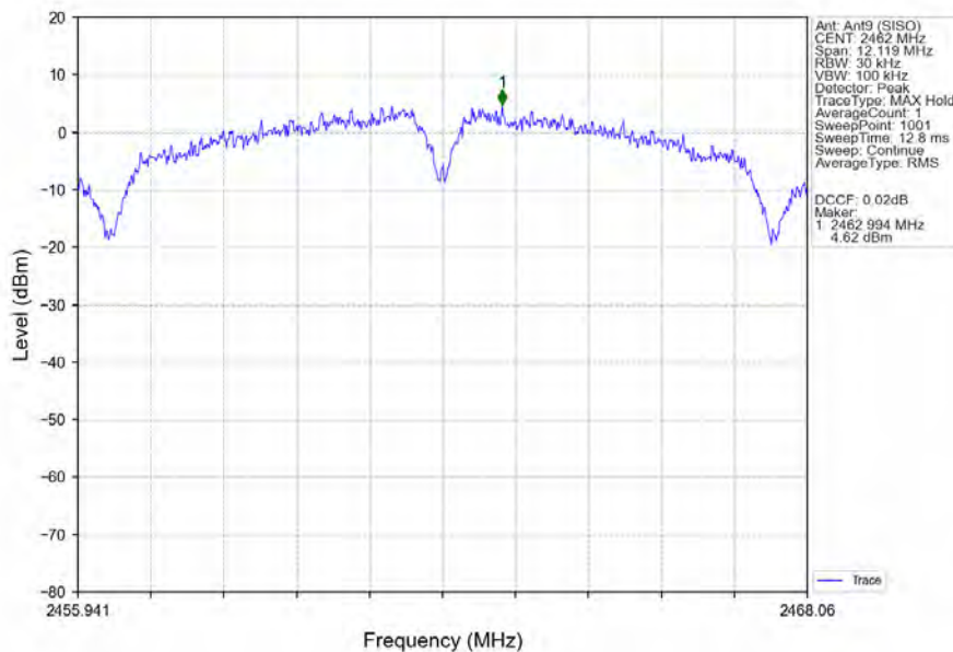
802.11b_HCH_2462MHz_Ant9 (SISO)_NTNV
