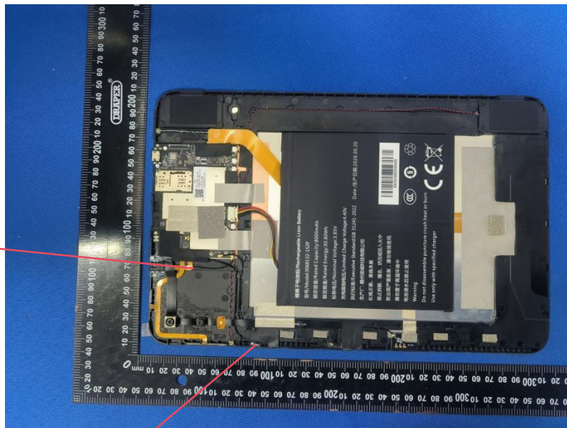
LTE 4G DIV Antenna
