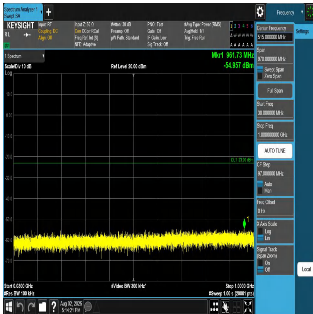
Band25-20MHz-QPSK-26365-1RB#0-30~1000-PASS
