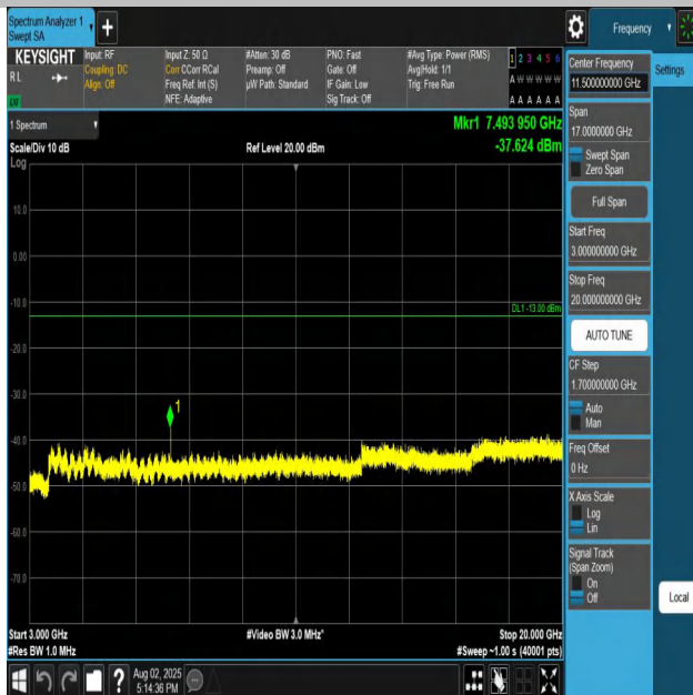
Band25-20MHz-QPSK-26365-1RB#0-3000~20000-PASS
