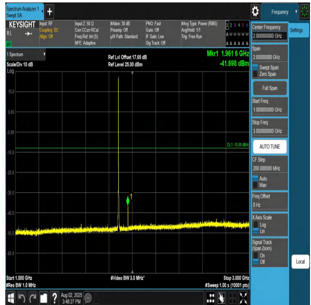
Band25-3MHz-QPSK-26365-1RB#0-1000~3000-PASS
