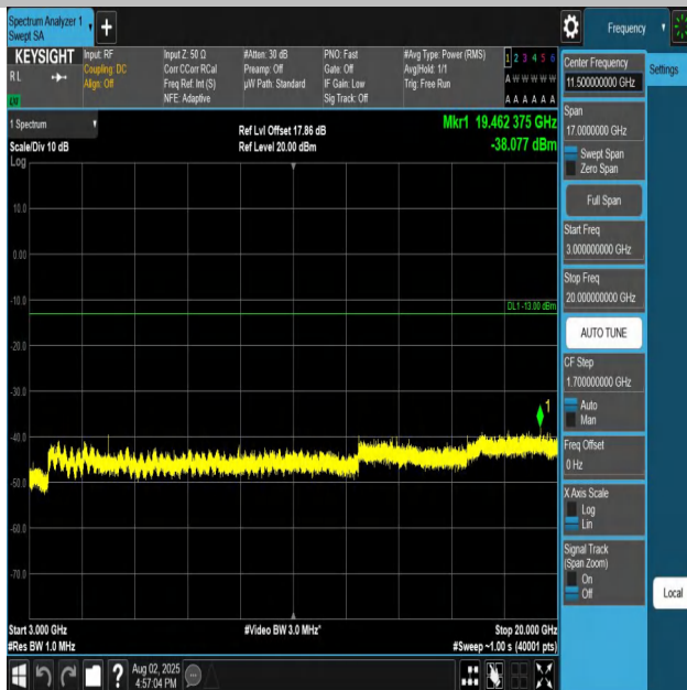
Band25-15MHz-QPSK-26115-1RB#0-3000~20000-PASS
