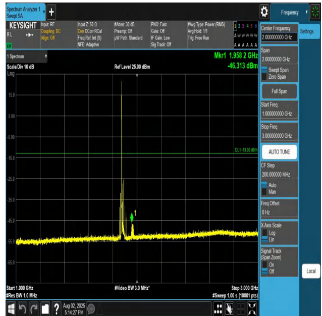
Band25-20MHz-QPSK-26365-1RB#0-1000~3000-PASS
