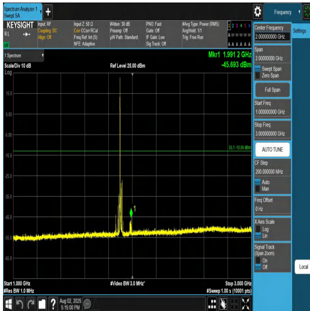
Band25-20MHz-QPSK-26590-1RB#0-1000~3000-PASS
