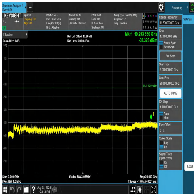
Band25-10MHz-QPSK-26365-1RB#0-3000~20000-PASS
