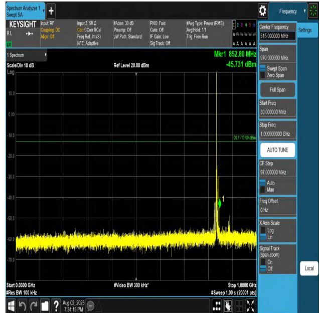
Band26(824-849)-10MHz-QPSK-26990-1RB#0-30~1000-P ASS
