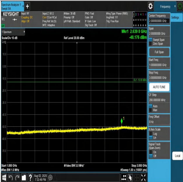
Band26(824-849)-10MHz-QPSK-26915-1RB#0-1000~300 0-PASS
