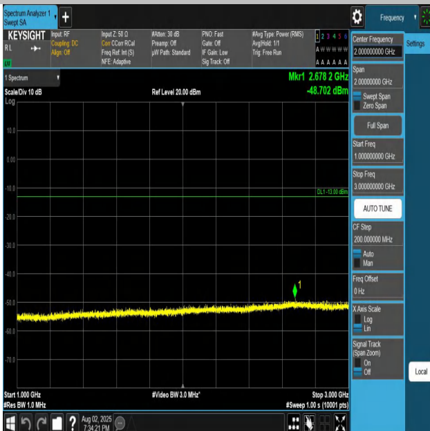
Band26(824-849)-10MHz-QPSK-26990-1RB#0-1000~300 0-PASS
