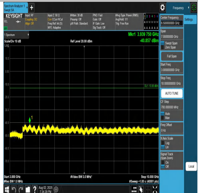
Band26(824-849)-10MHz-QPSK-26990-1RB#0-3000~100 00-PASS
