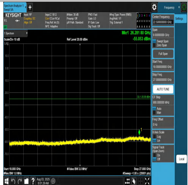
Band41-20MHz-QPSK-41490-1RB#0-18000~27000-PASS
