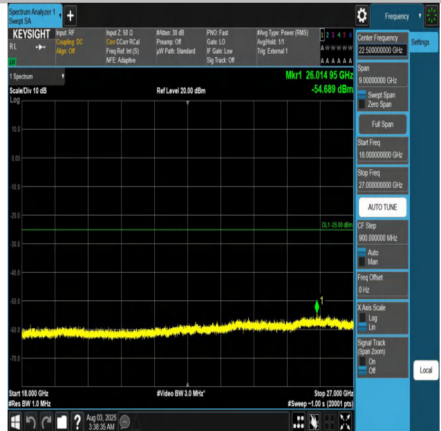
Band41-5MHz-QPSK-41565-1RB#0-18000~27000-PASS
