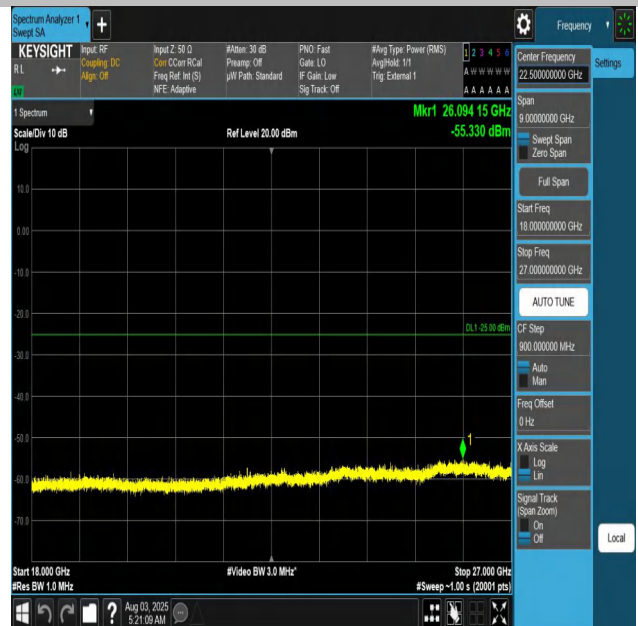
Band41-15MHz-QPSK-39725-1RB#0-18000~27000-PASS
