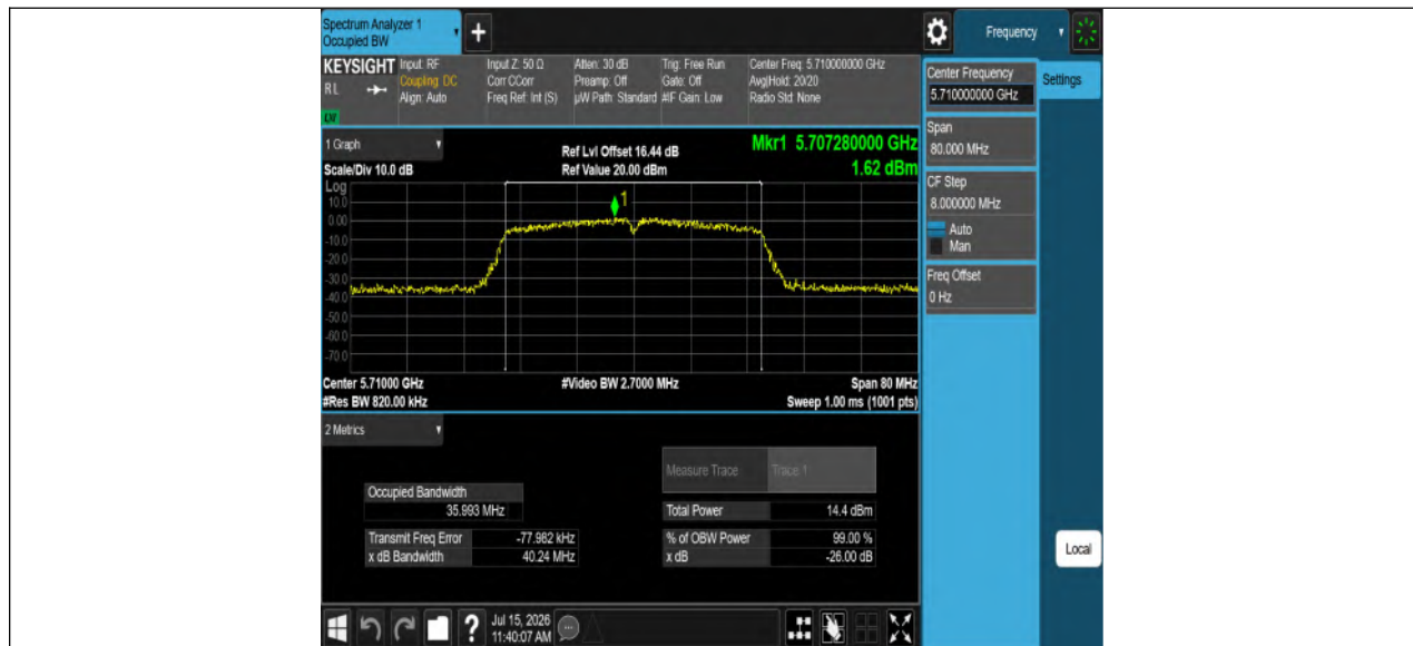
11N40MIMO_Ant2_5710
