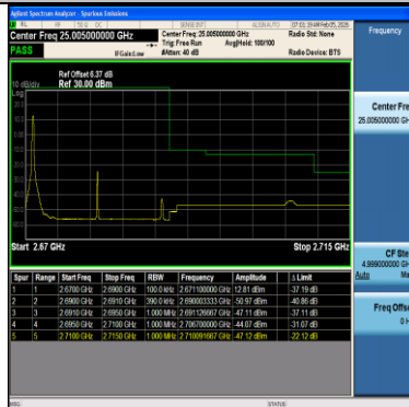
Band41-20MHz-QPSK-41490-1RB#99-PASS
