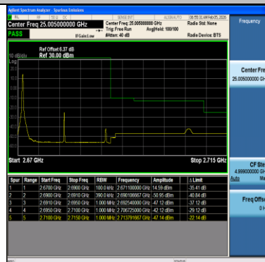
Band41-20MHz-QPSK-41490-1RB#0-PASS
