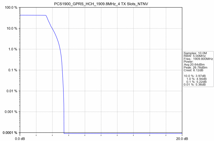
PCS1900_GPRS_HCH_1909.8MHz_4 TX Slots_NTNV
