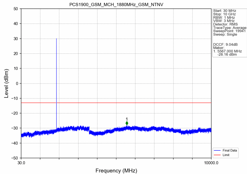
PCS1900_GSM_MCH_1880MHz_GSM_NTNV
