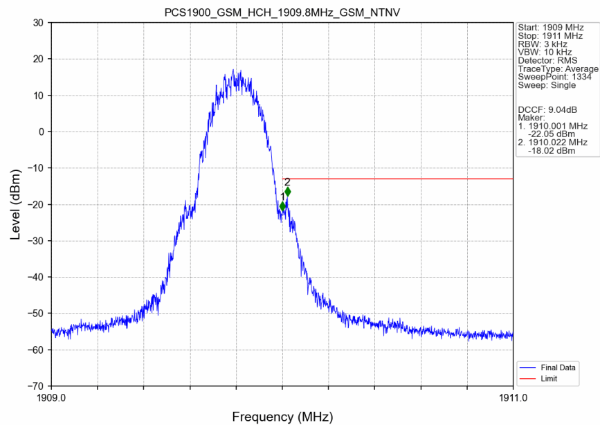
PCS1900_GSM_HCH_1909.8MHz_GSM_NTNV
