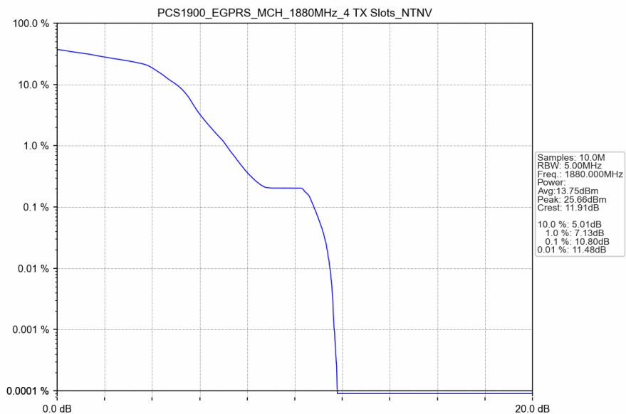
PCS1900_EGPRS_MCH_1880MHz_4 TX Slots_NTNV
