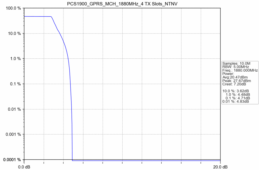
PCS1900_GPRS_MCH_1880MHz_4 TX Slots_NTNV
