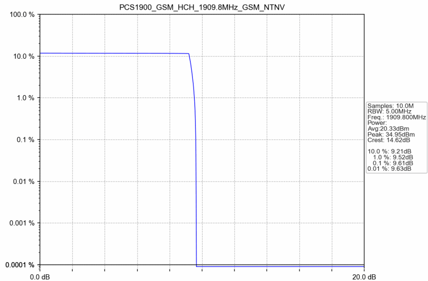
PCS1900_GSM_HCH_1909.8MHz_GSM_NTNV
