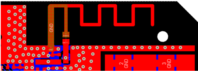
PIFA antenna
