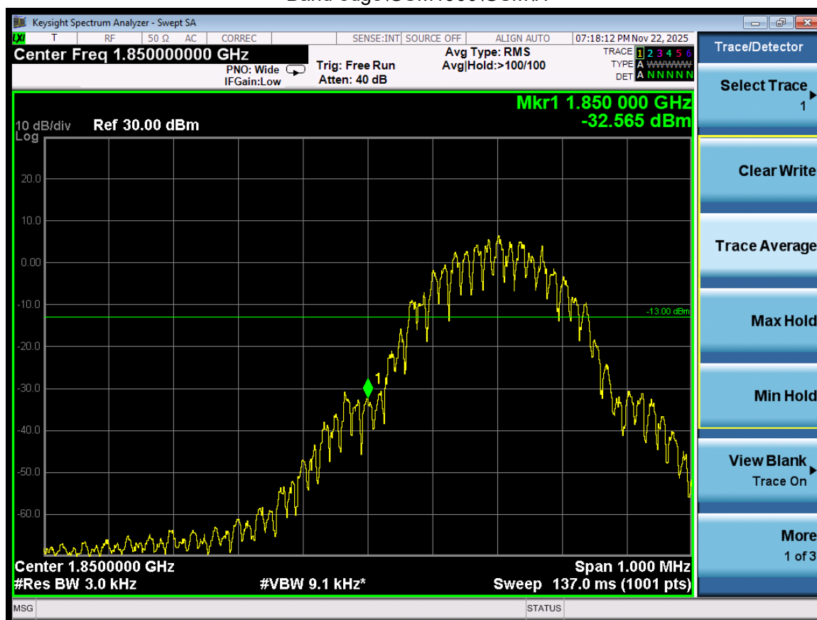
Band edge\GSM1900\GSM L
