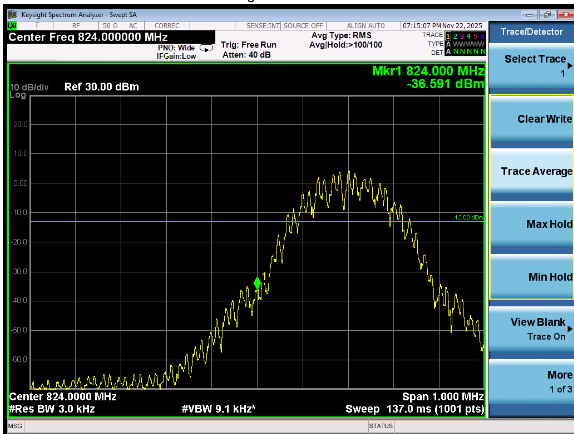
Band edge\GSM850\EGPRS\L
