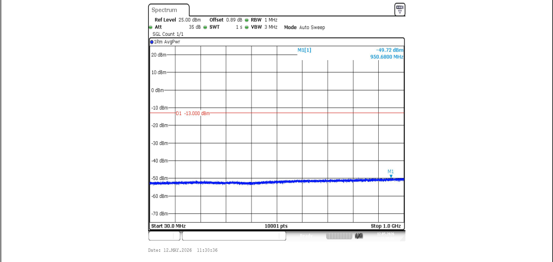
Band2-9400-1-30~1000MHz-PASS
