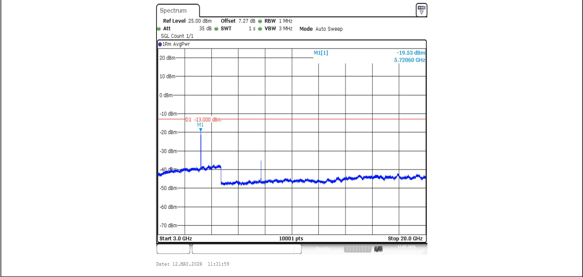
Band2-9538-1-3000~20000MHz-PASS
