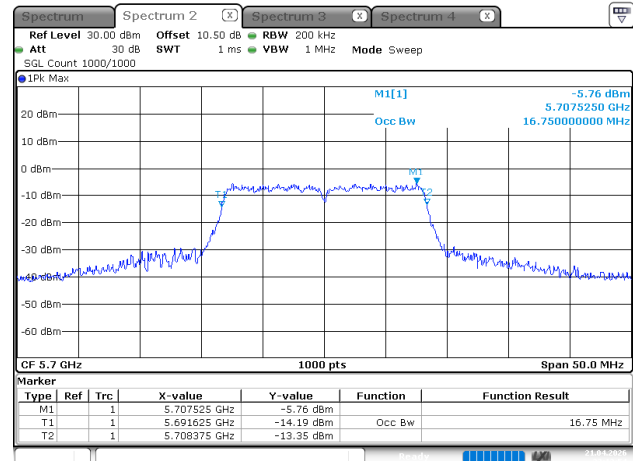
802.11a_5700MHz
