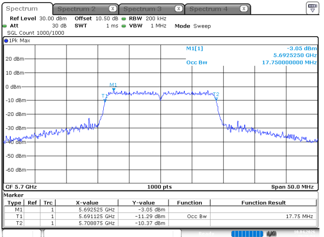
802.11ac20_5700MHz
