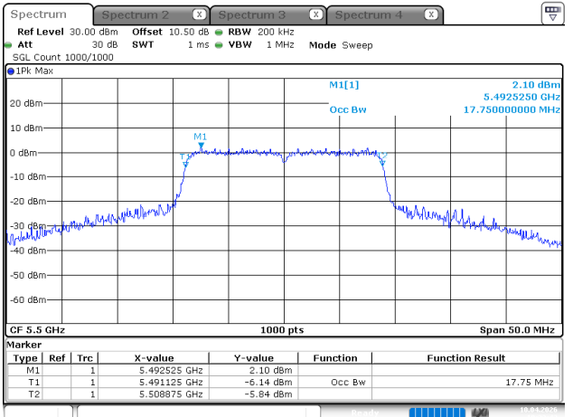
802.11ac20_5500MHz
