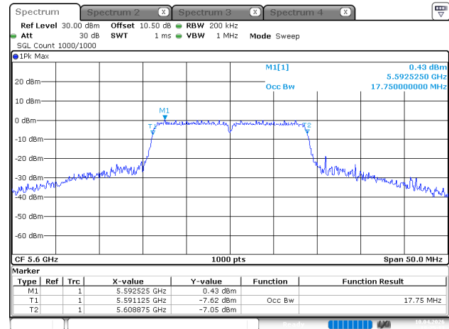
802.11ac20_5600MHz
