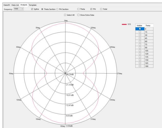
GPS(L1) Phi=0deg
