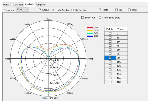
WIFI 2.4G/BT Theta=90deg
