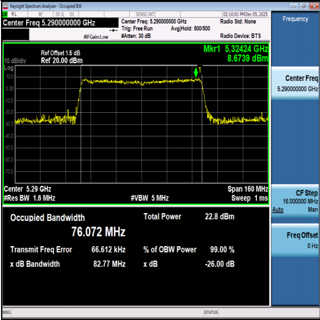
11AC80SISO-Ant1-5290
