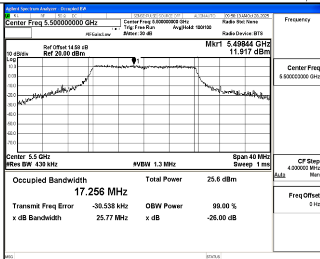
11N20MIMO Ant2 5500
