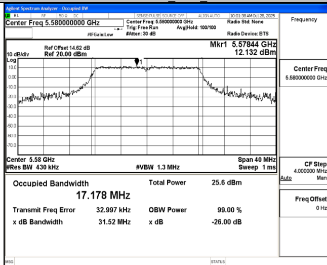
11N20MIMO Ant2 5580
