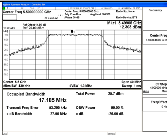
11N20MIMO Ant2 5500
