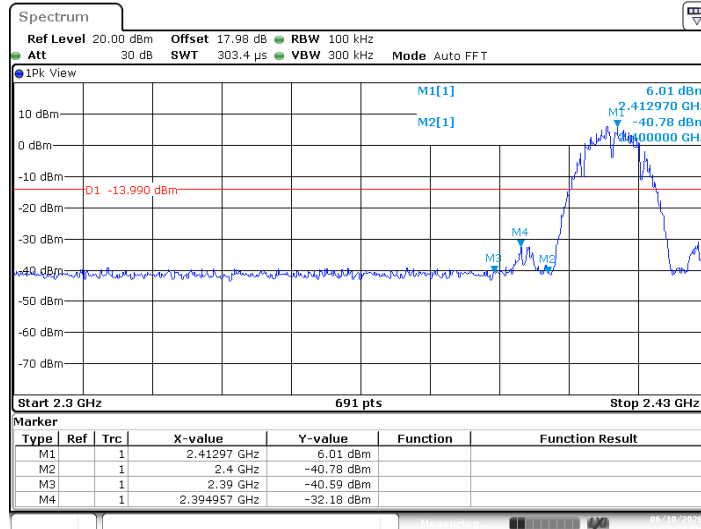
11B_Ant1_Low_2412
