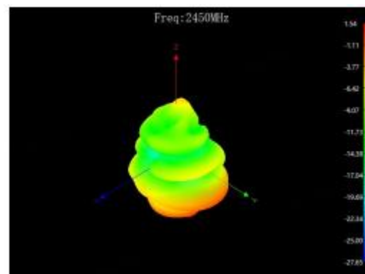
2500MHz 3D
