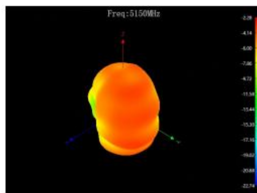
5450MHz 3D
