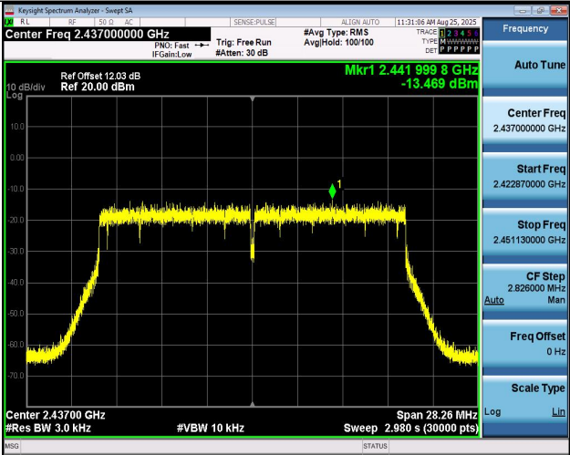
11BE20MIMO-Ant1-2437-PASS
