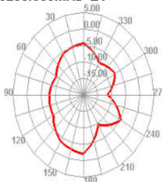
5250.000MHz E1
