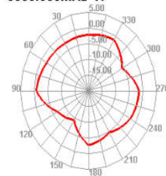
5850.000MHz H
