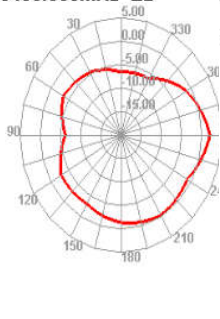
5450.000MHz E2
