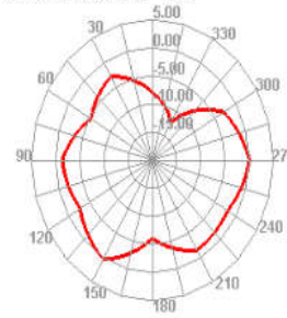
5650.000MHz E2
