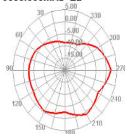
5550.000MHz E2
