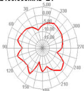
2400.000MHz E1
