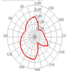
5350.000MHz E1
