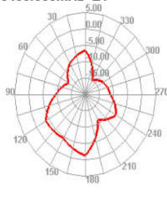
5450.000MHz E1
