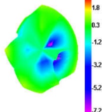
5850.000MHz E1
