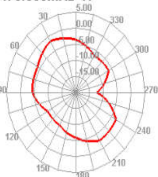
2475.000MHz H
