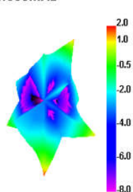
5450.000MHz E1
