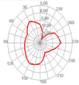
5650.000MHz E1
