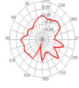
2450.000MHz E2
