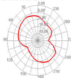
2500.000MHz H
