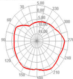
5150.000MHz E2
