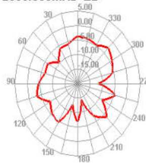
2500.000MHz E2
