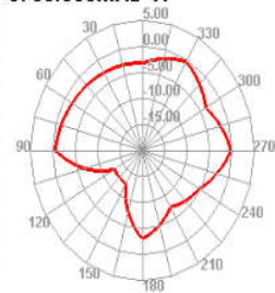
5750.000MHz E2
