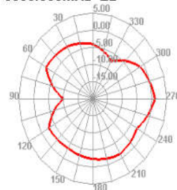
5350.000MHz E2
