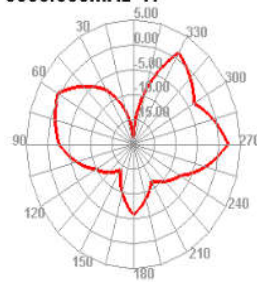
5550.000MHz H
