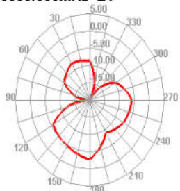
5550.000MHz E1
