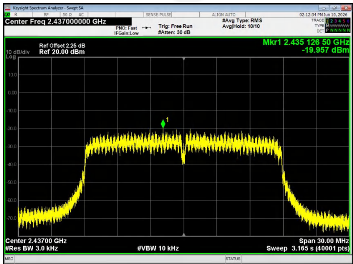
802.11n20 - CH06
