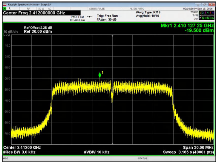
802.11n20 - CH01
