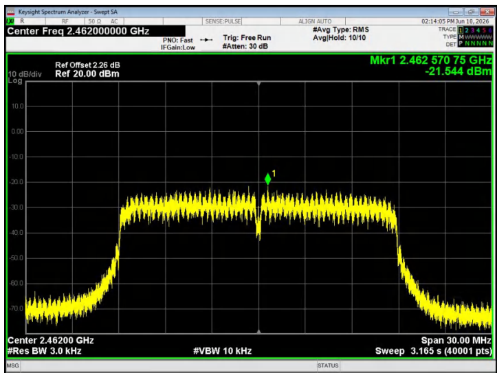
802.11n20 - CH11
