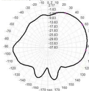
2450.0MHz Total(E1-XZ), Max= 2.17dBi
