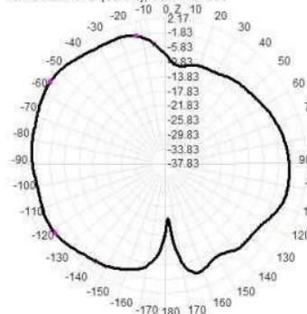
2450.0MHz Total(E2-YZ), Max= 1.26dBi
