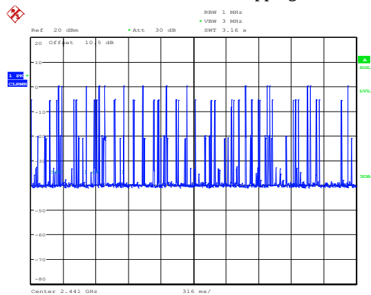
2EDR_DH3_Hopping
