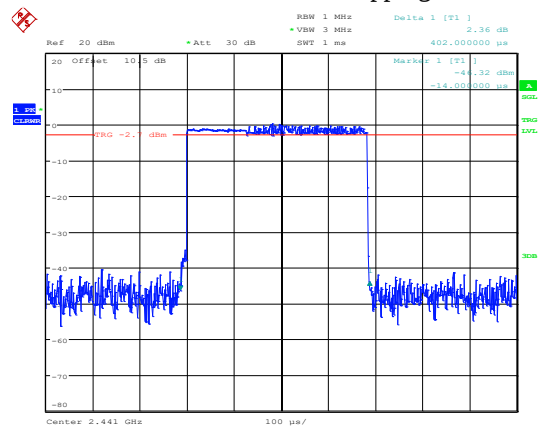
2EDR_DH1_Hopping
