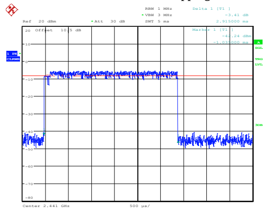
2EDR_DH5_Hopping
