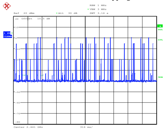
2EDR_DH5_Hopping
