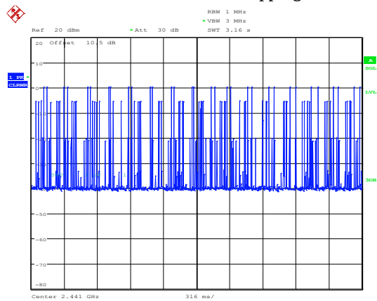
2EDR_DH1_Hopping
