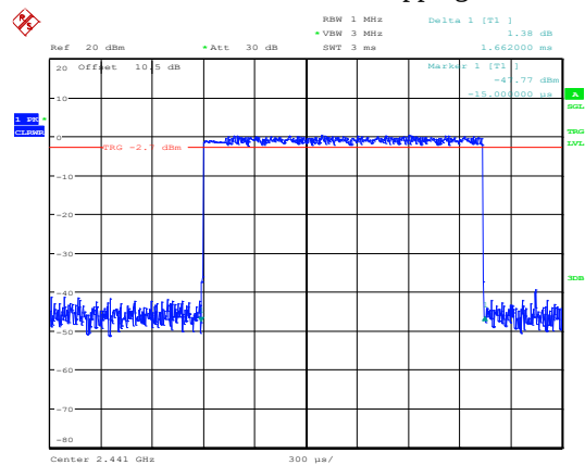
2EDR_DH3_Hopping
