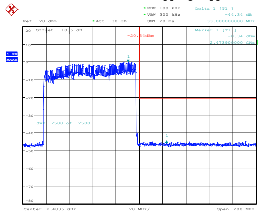
2EDR_DH1_Hopping_Upper
